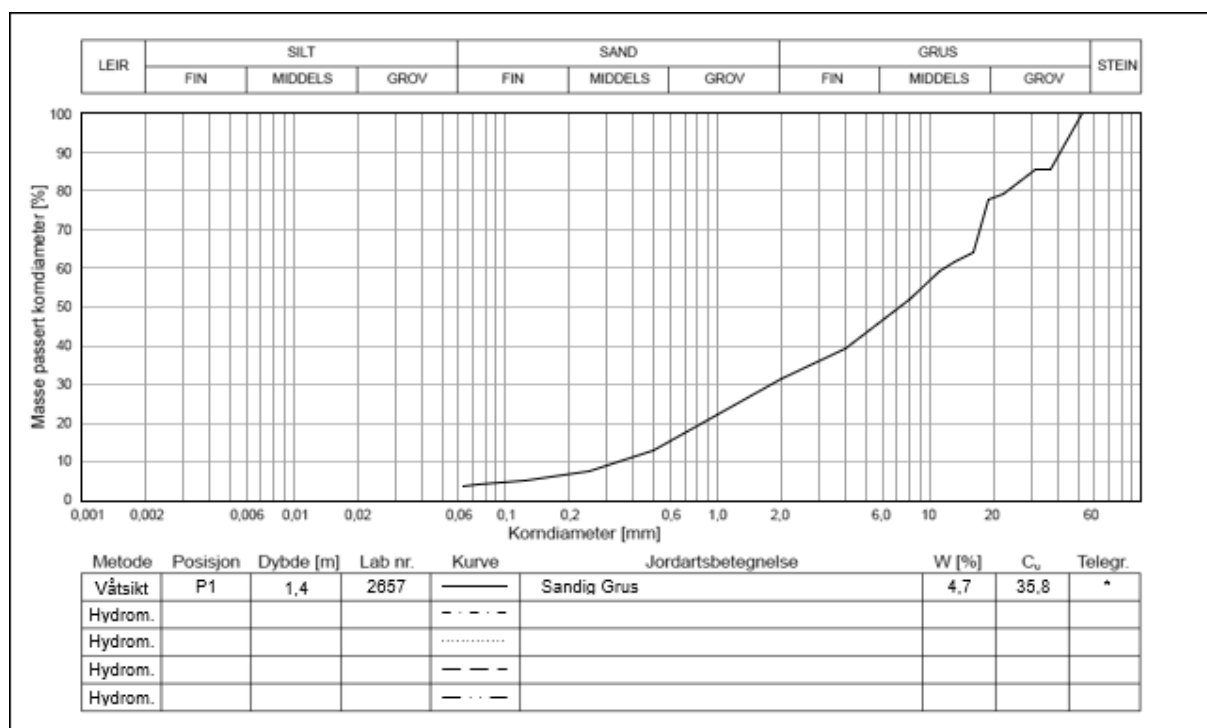
Figur 4 Kornfordeling utført av Norconsults laboratoriet i Molde.
