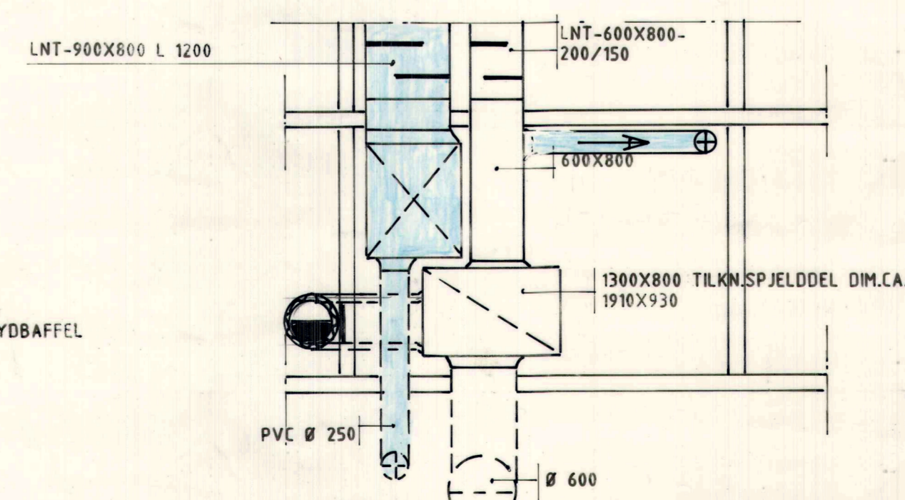
SNITT 2:2
