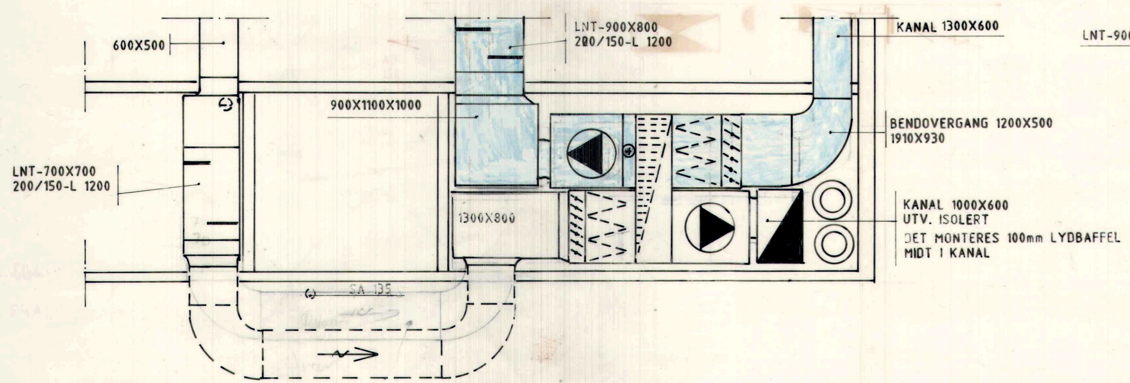
SNITT 1:1
