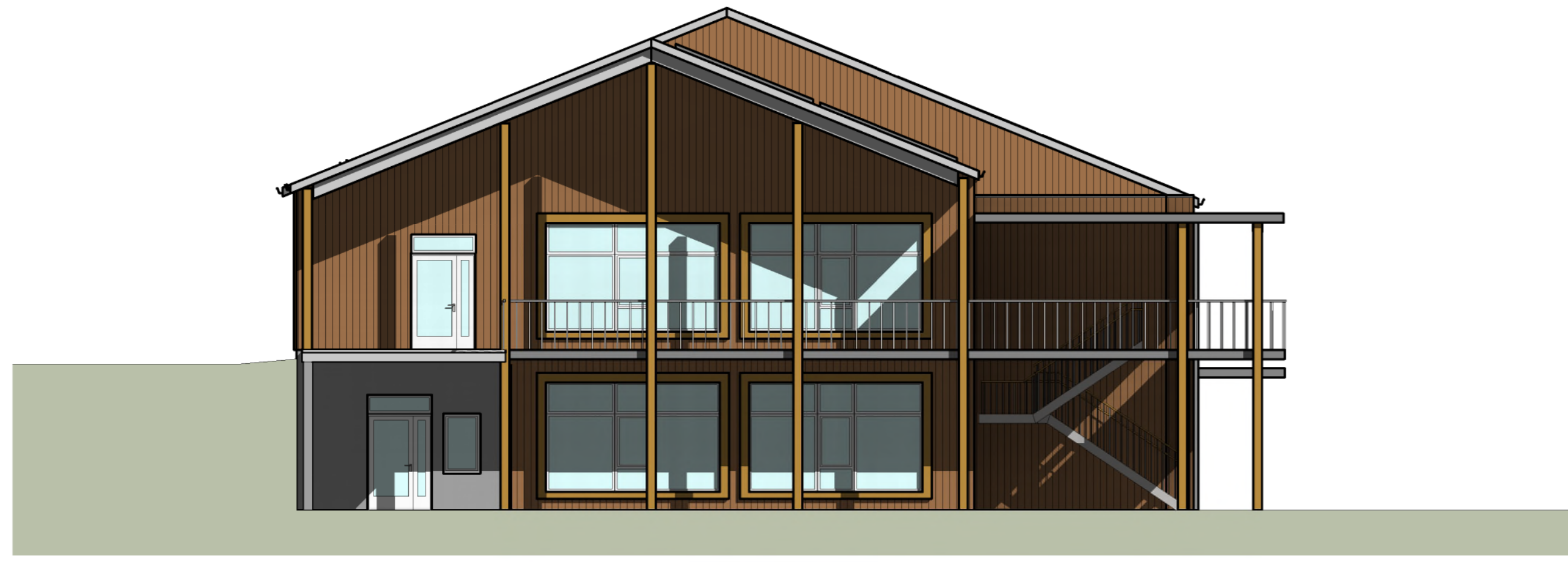
Fasade Vest 1:100
