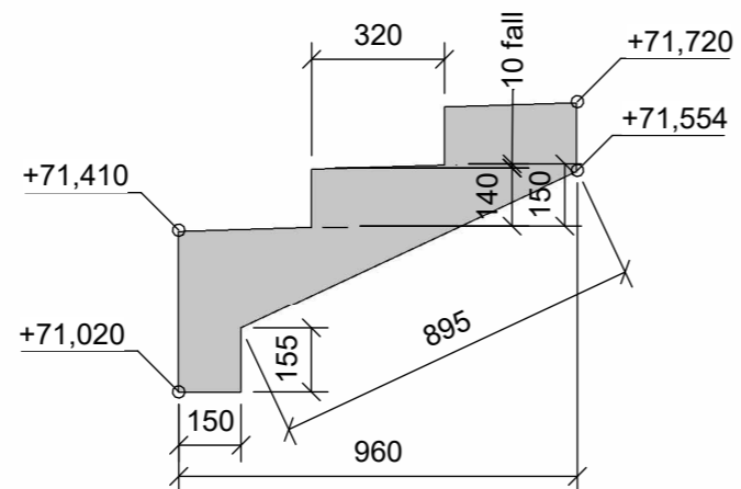
Snitt 301 1 : 20
