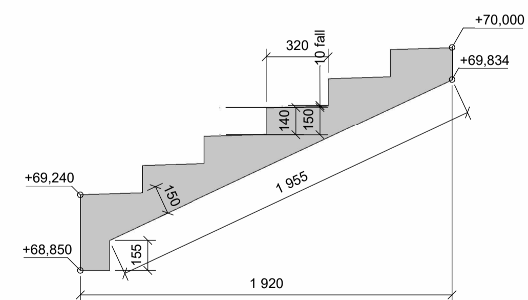
Snitt 202 1 : 20
