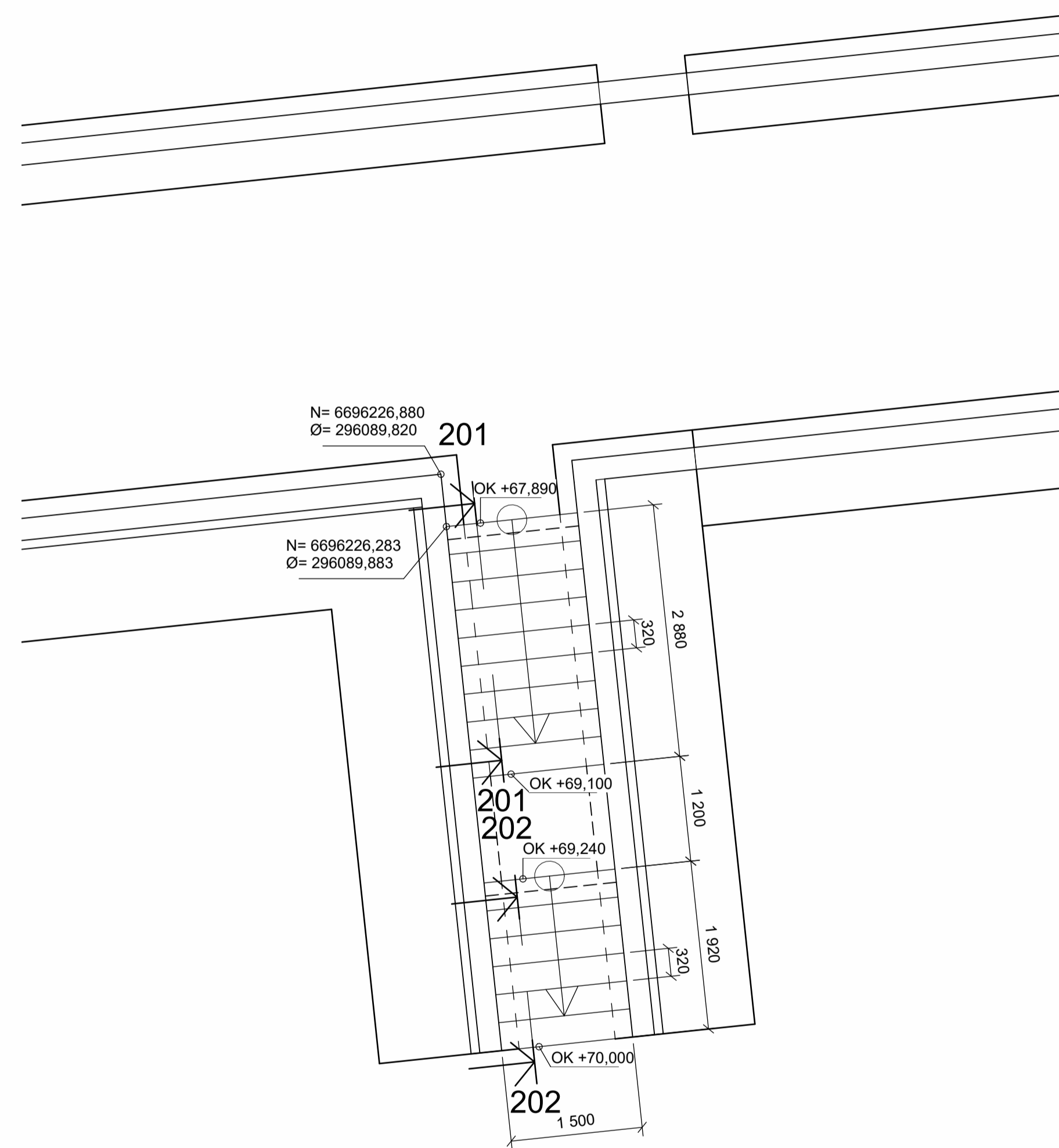
Plan Trapp 2 1 : 50
