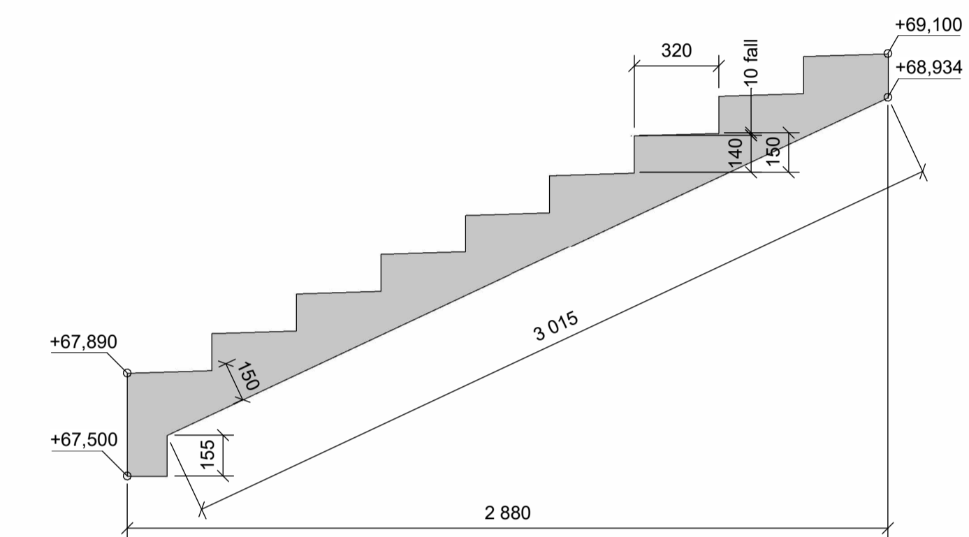
Snitt 201 1 : 20
