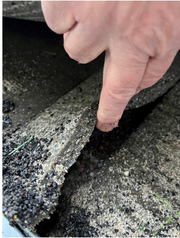
Figur 9 og 10 Fra hjørnet i nord-vest. Eksisterende kunstgress med pad. Ligger mot dreneringsrenne på kortsiden mot nord. Kunstgress system: Polytan, Liga Turf RS Pro II Cool Plus SBR 40mm med pad Recticel 14 mm. Hele systemet skal fjernes og avhendes ihht Forurensningsforskriften.
