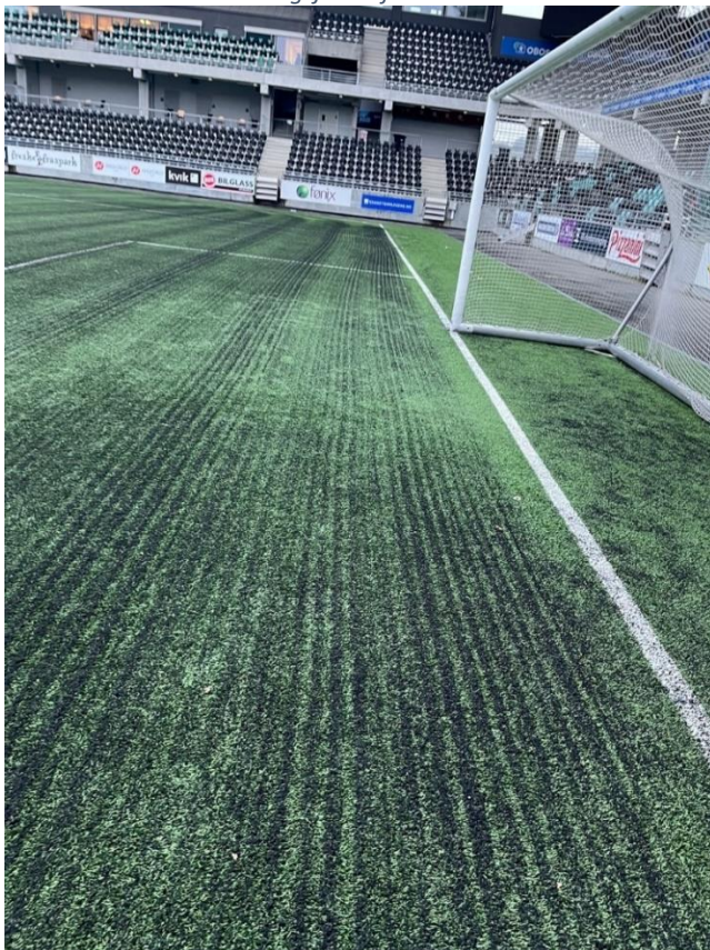
Figur 11 Fra kortsiden mot nord. Her er det 3m med kunstgress fram til dreneringsrennen. Deretter 3,66m med asfalt som fjernes og rør til vanningsanlegget legges. Asfalten erstattes med kunstgress.
