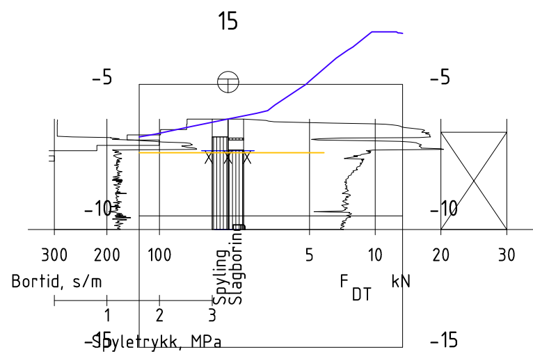
Profil D-D
