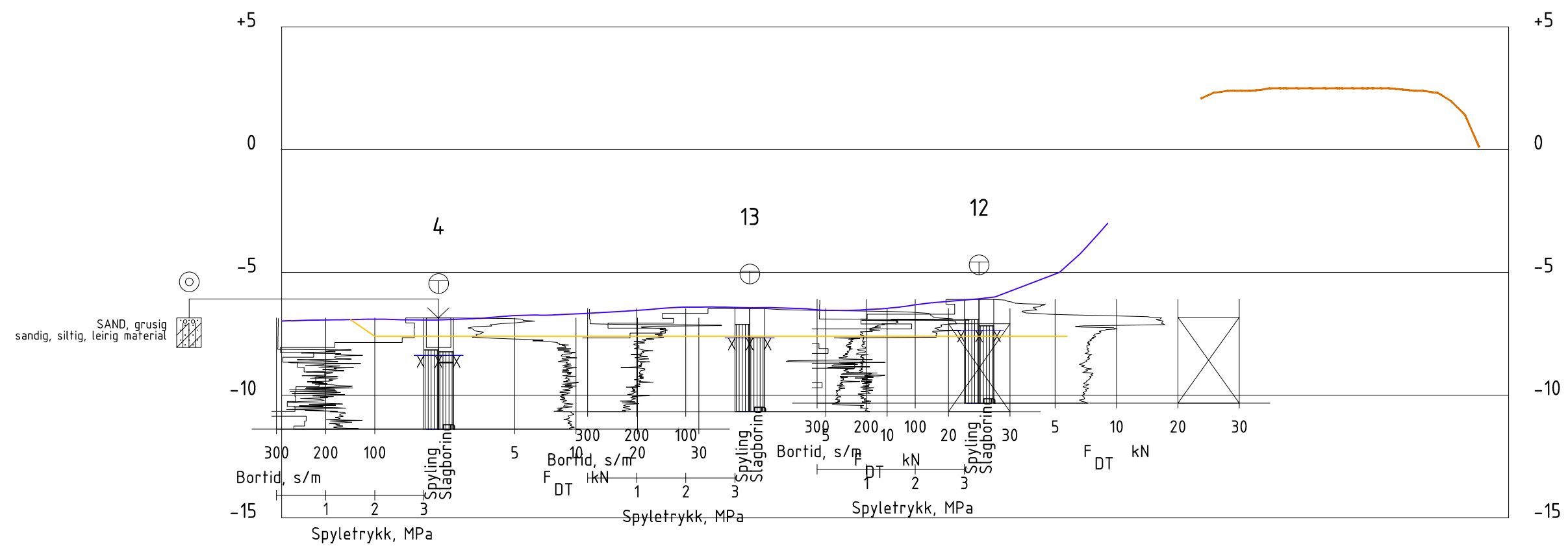
Profil B-B
