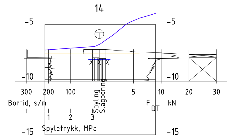
Profil F-F
