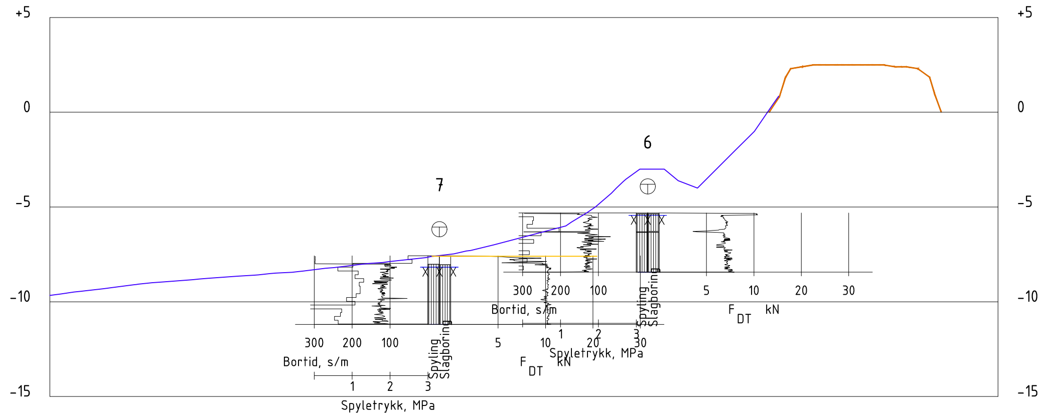
Profil G-G
