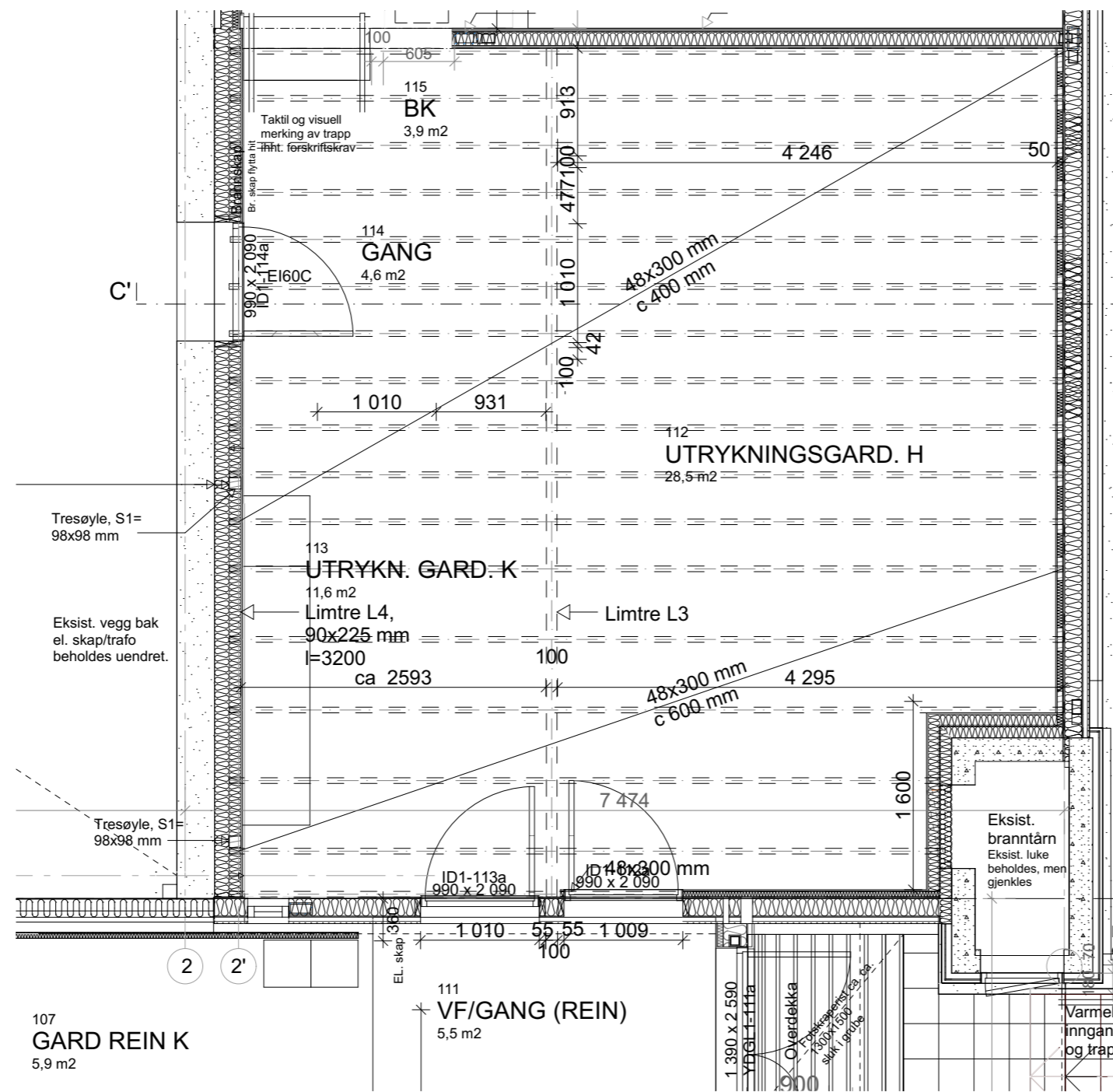
Bjelkelag over 1. etasje - eksisterende energisentral
