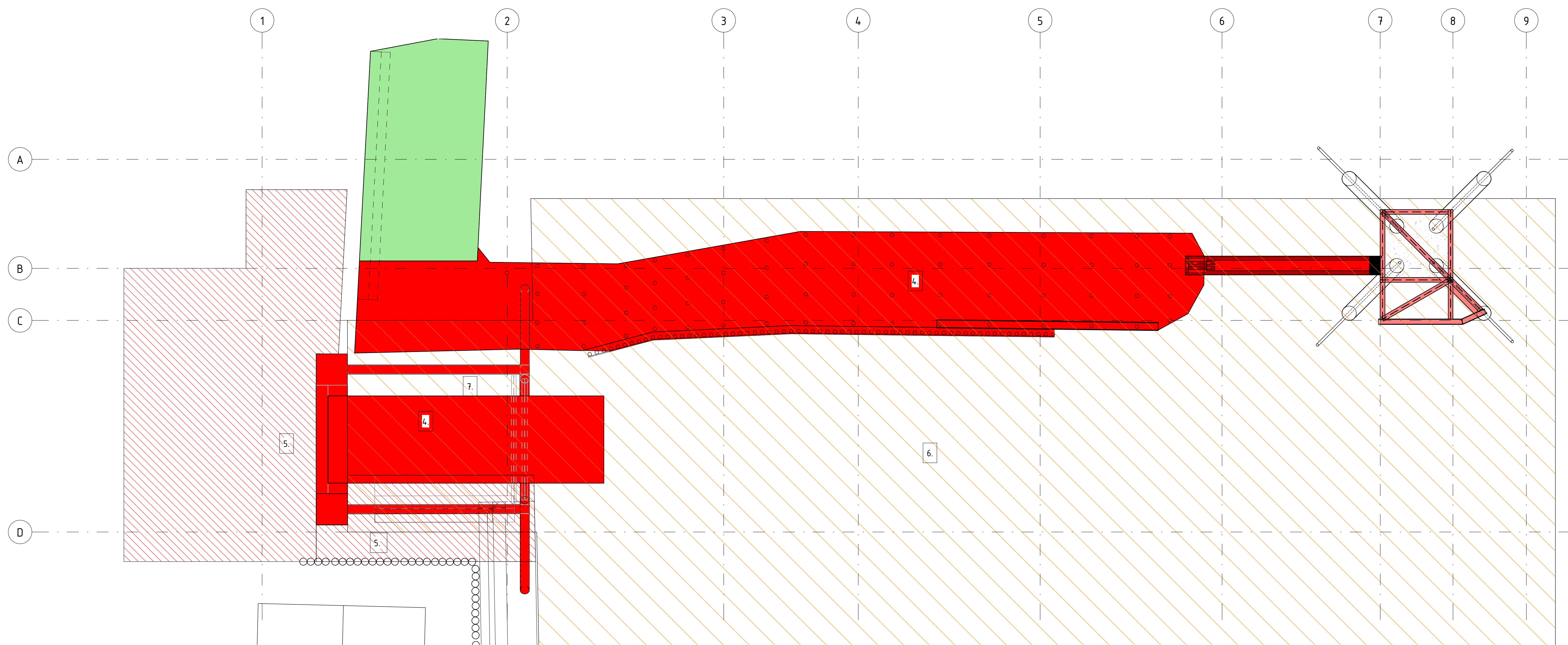
Fase 2 - del 1 - Stenøpeperiode 1 : 100
