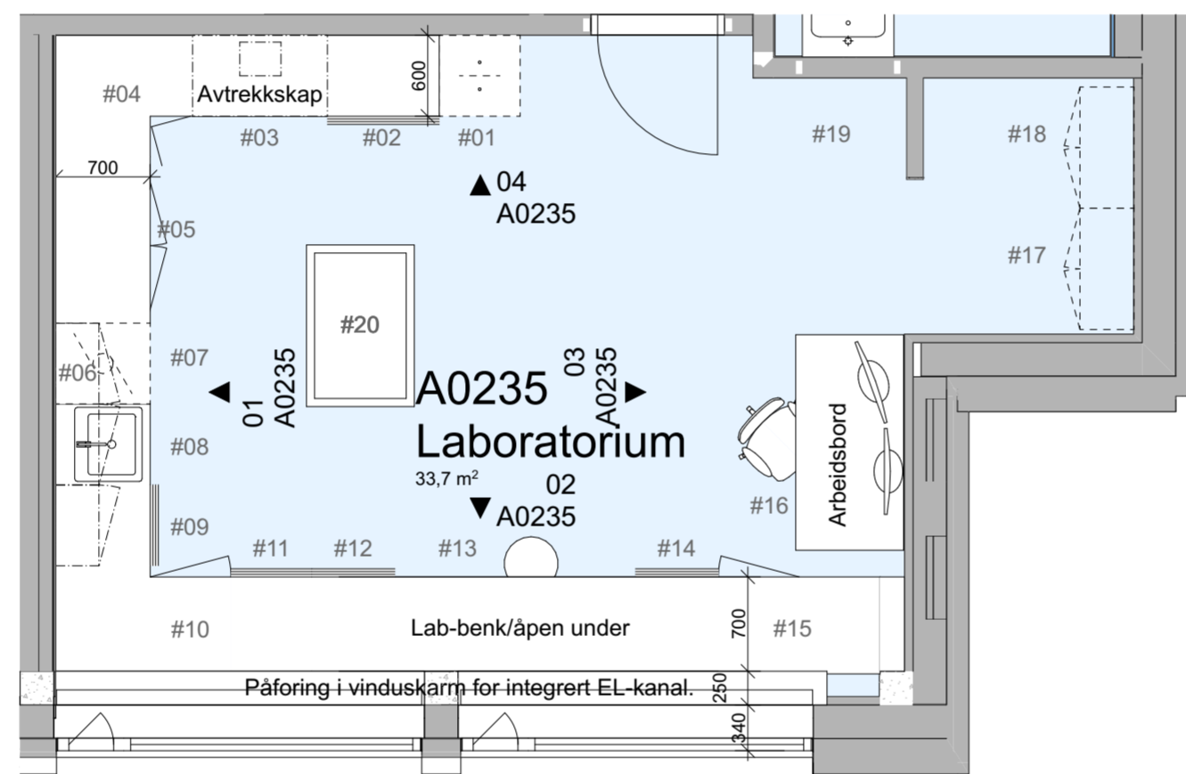
Møblering E-02 1:50
