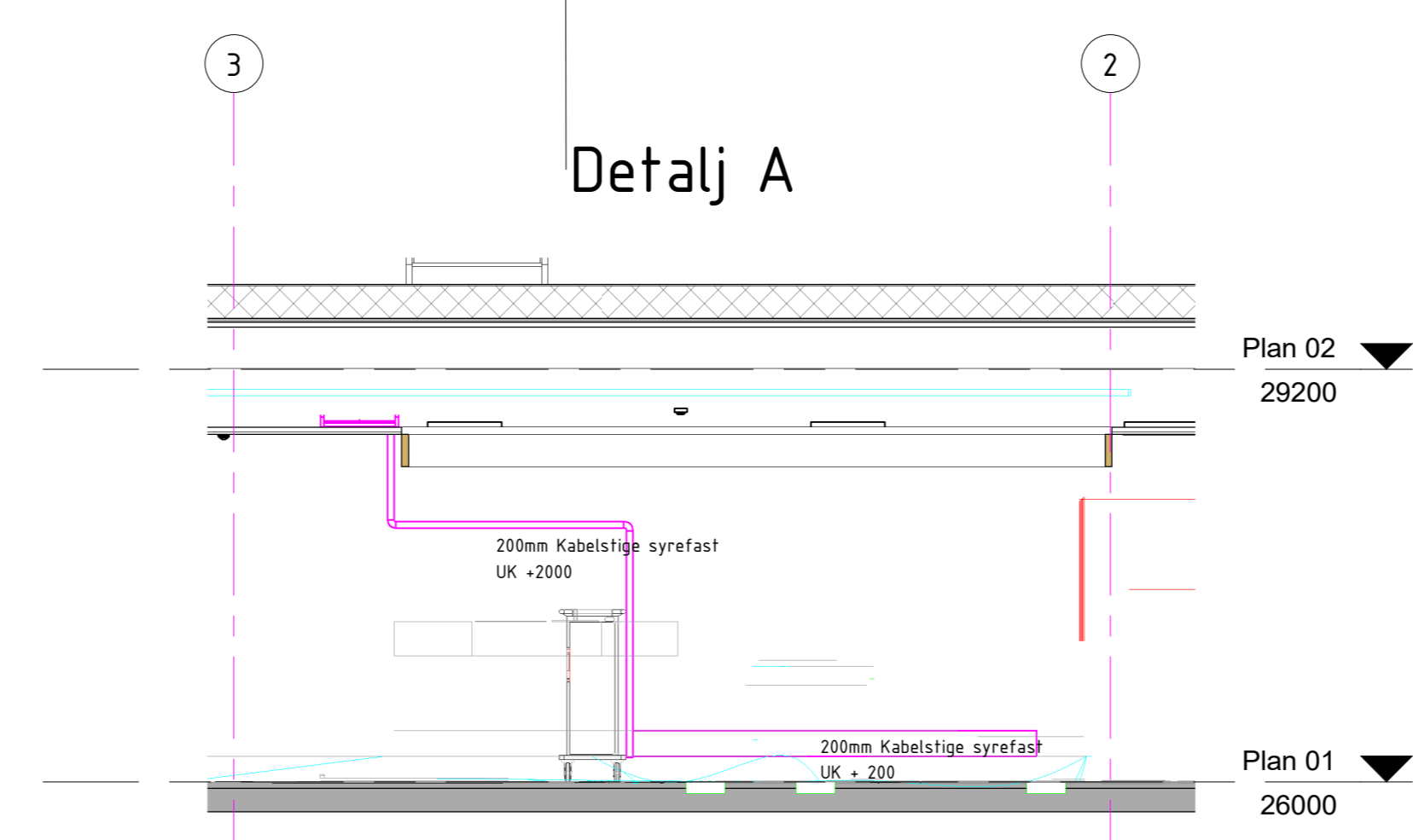
Detalj føringer til kokesone 1:50
