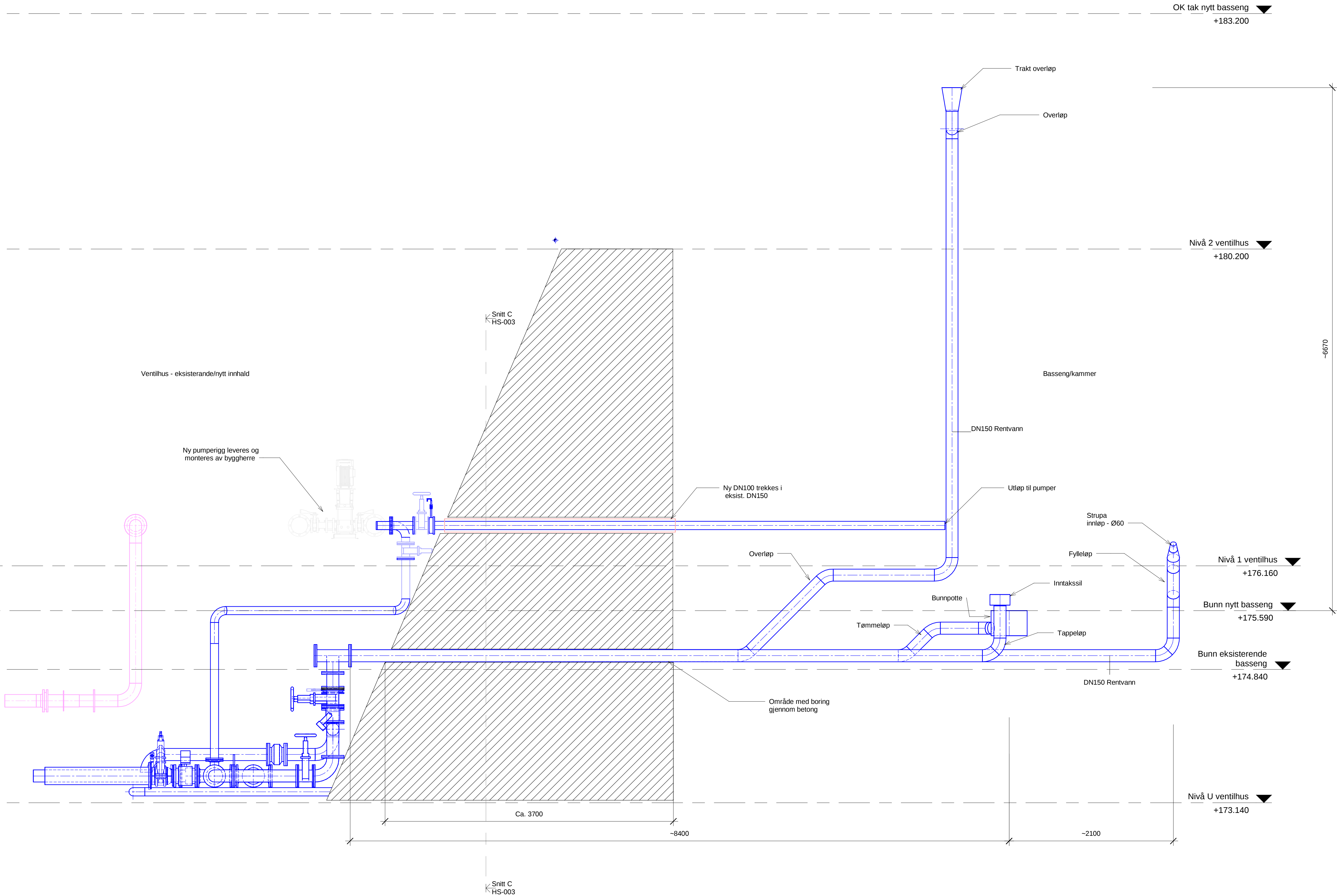
Snitt B 1 : 25
