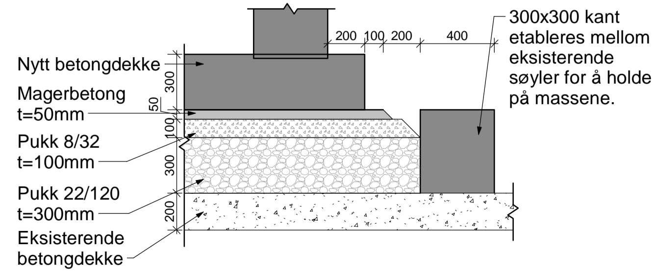
Lagoppbygging UK nytt basseng 1 : 20
