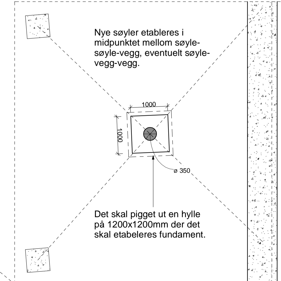
Plassering nye søyler 1 : 50
