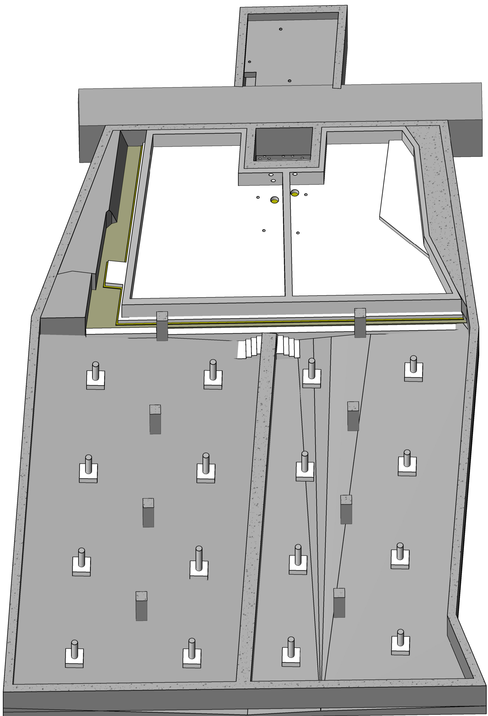
3D Underetasje
