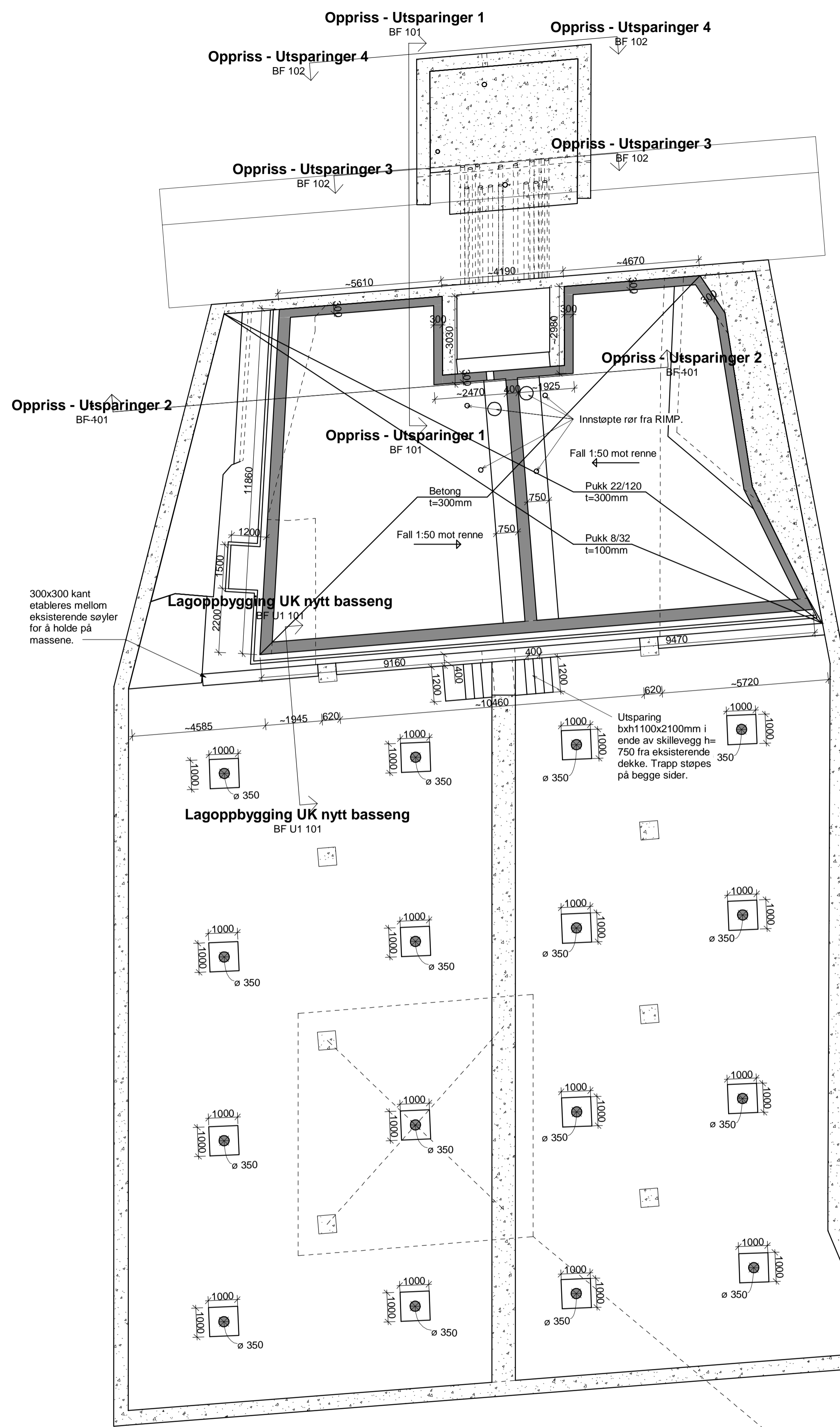
Plan - Underetasje 1 : 100
