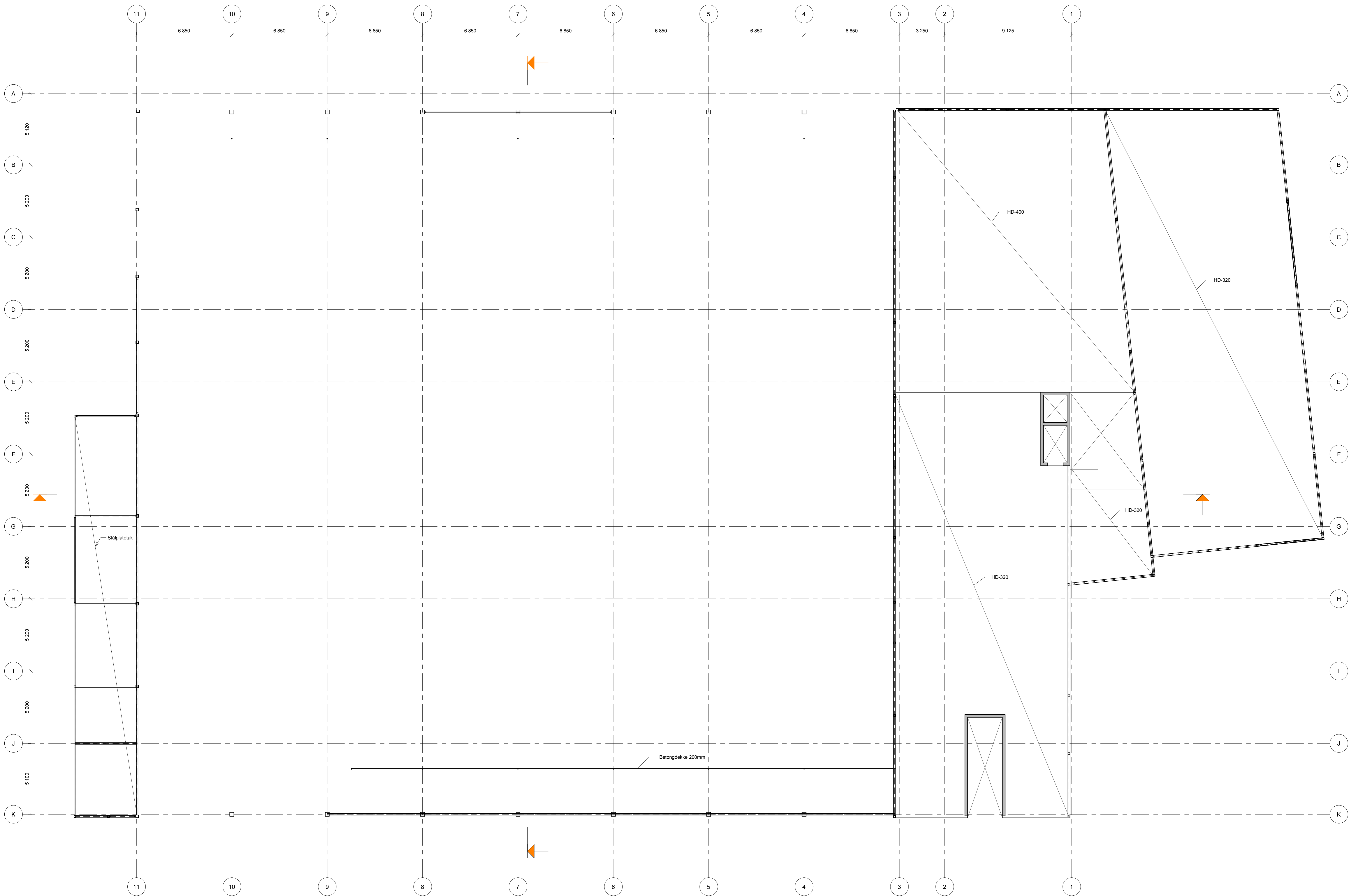
DEKKE OVER 01 1 : 100
