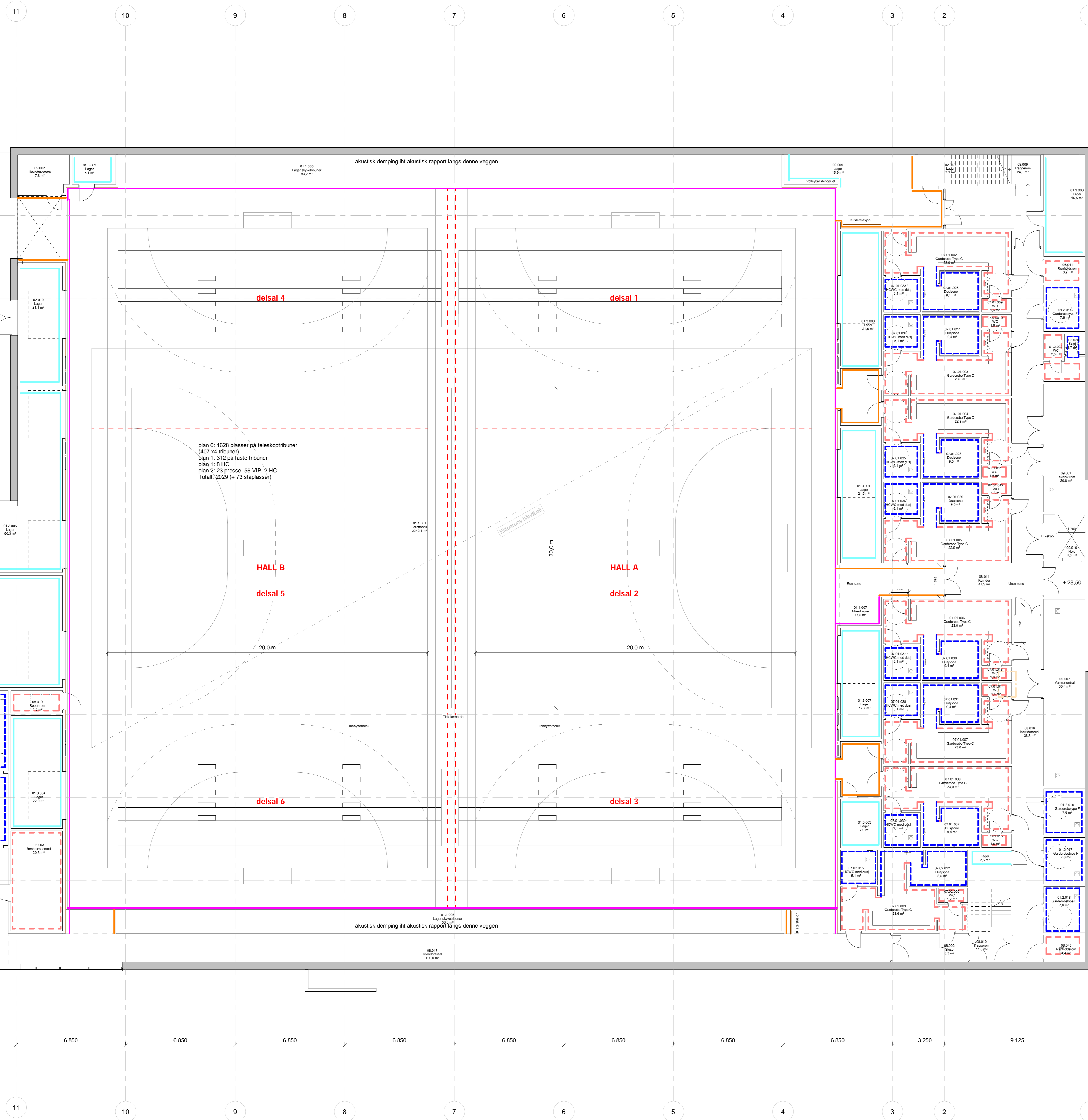
Veggplan-00 1 : 100
