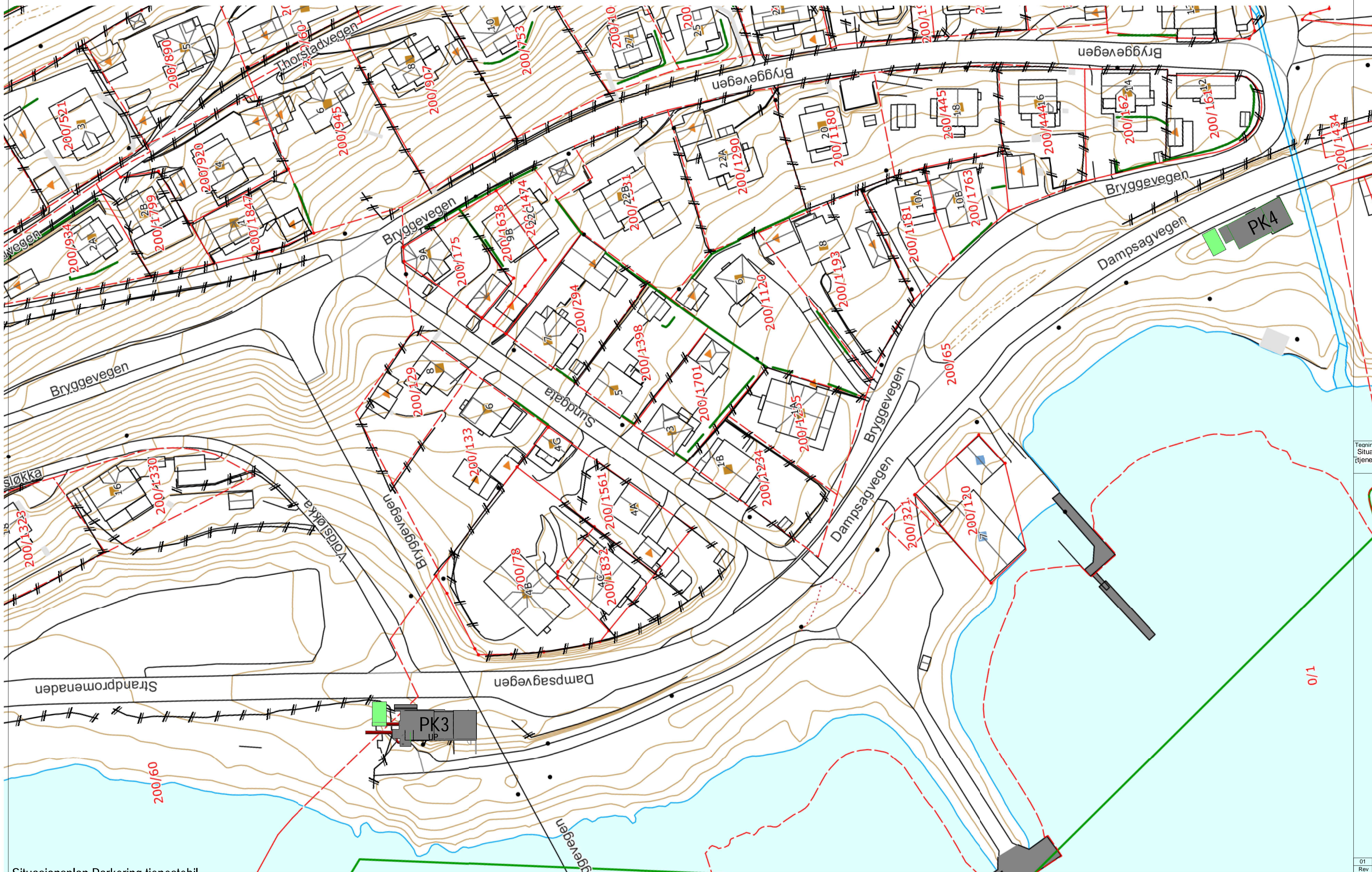
Situasjonsplan Parkering tjenestebil 1 : 500
