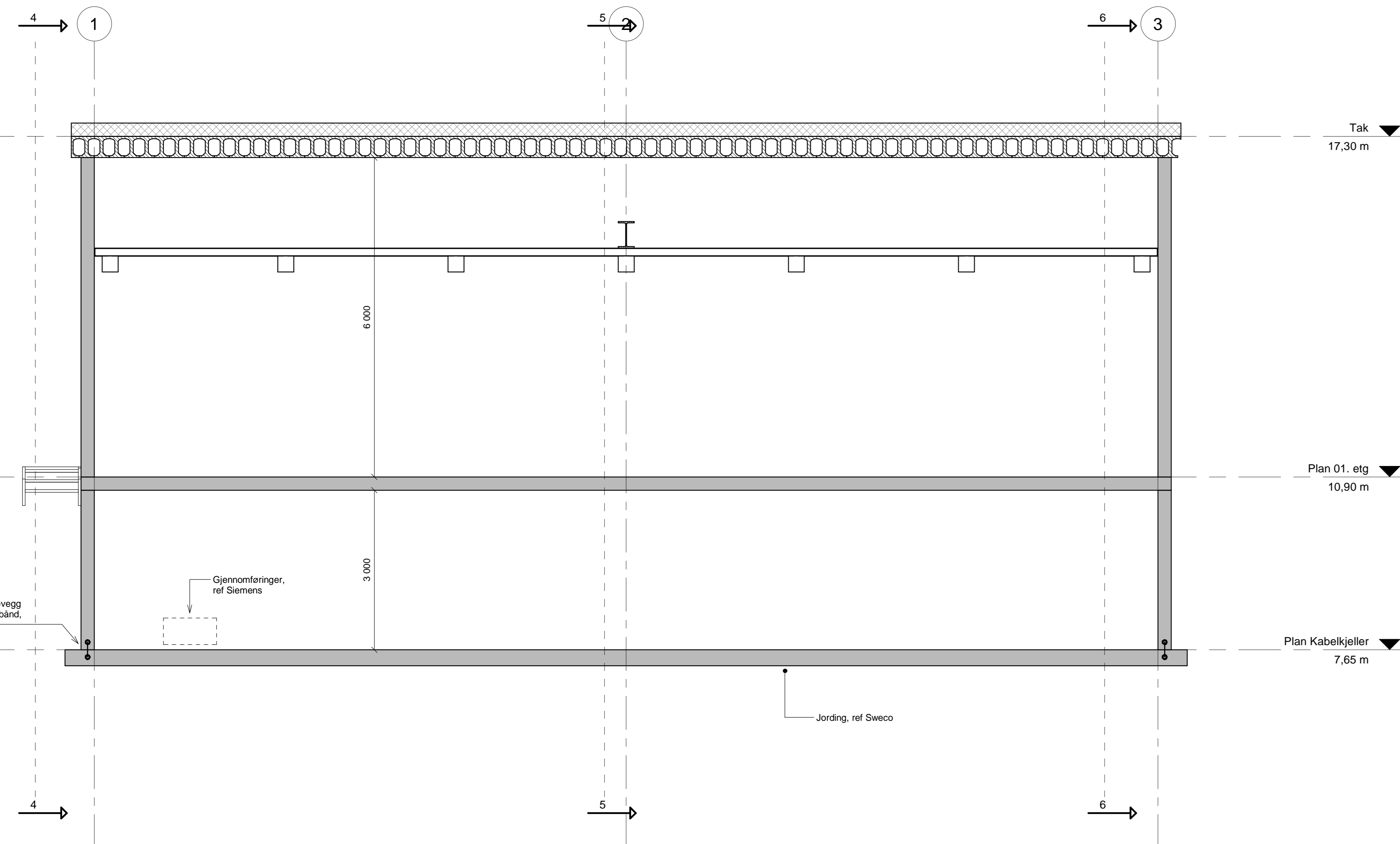
SNITT 3 1 : 50
