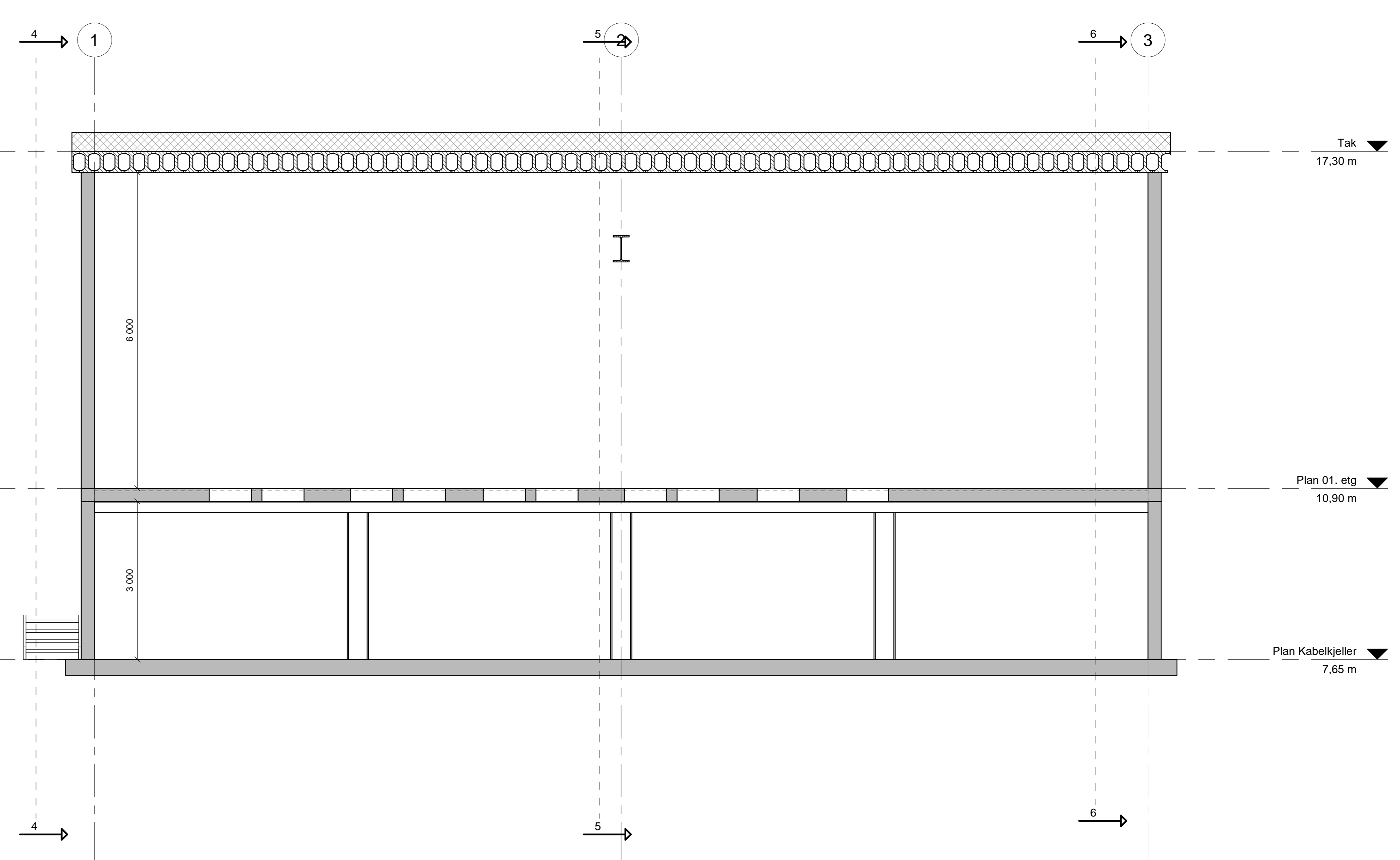
SNITT 2 1 : 50
