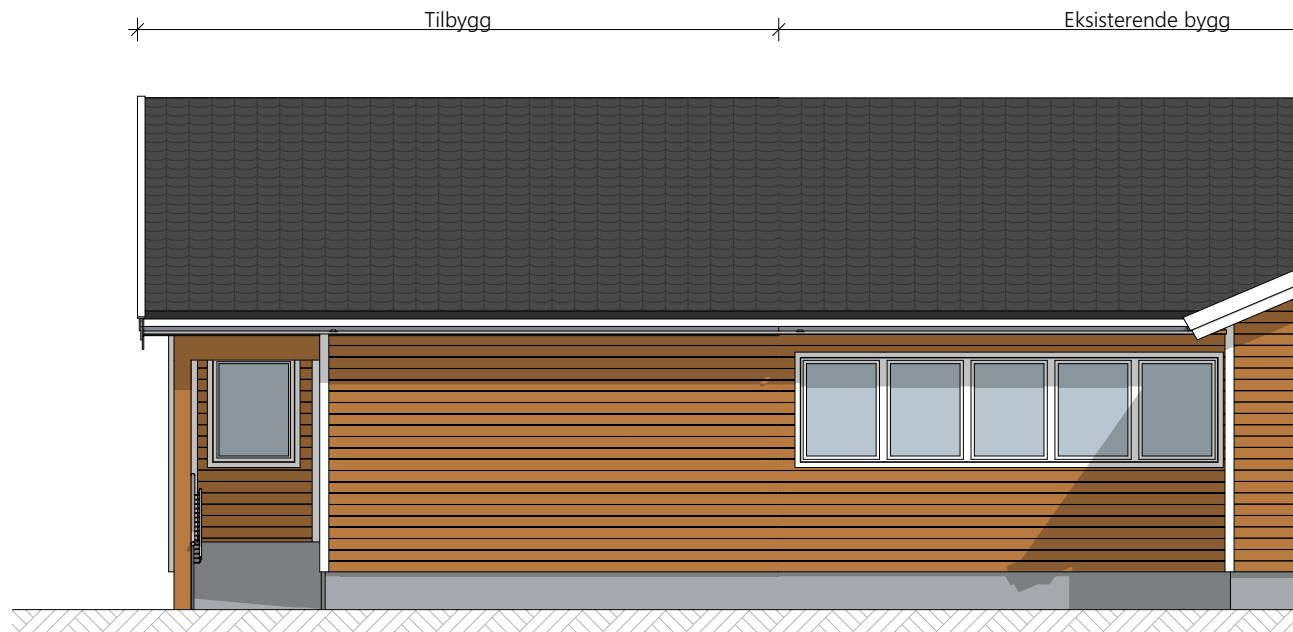
Fasade 1 1:100
