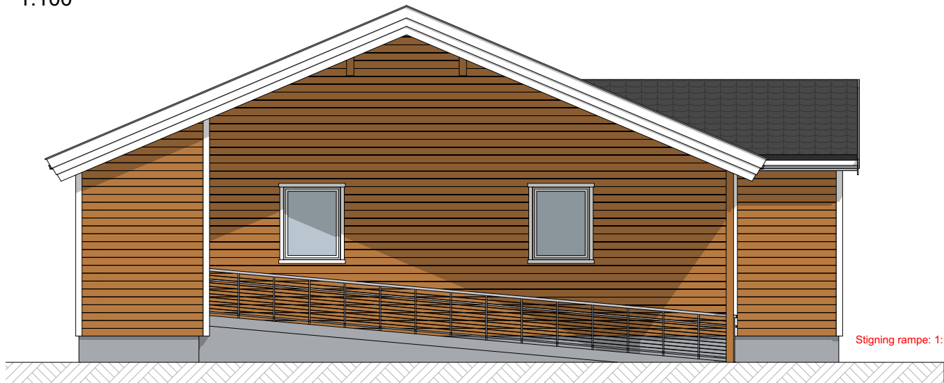
Fasade 3 1:100
