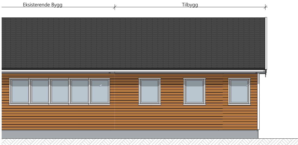
Fasade 2 1:100
