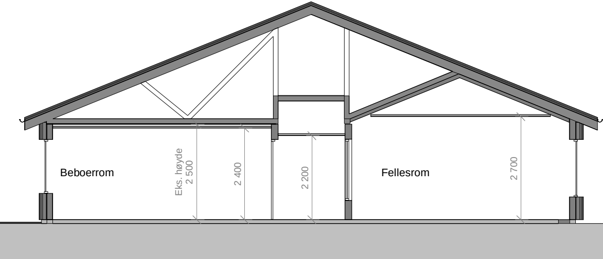
Snitt C-C Fjellblikk 1 1 : 100
