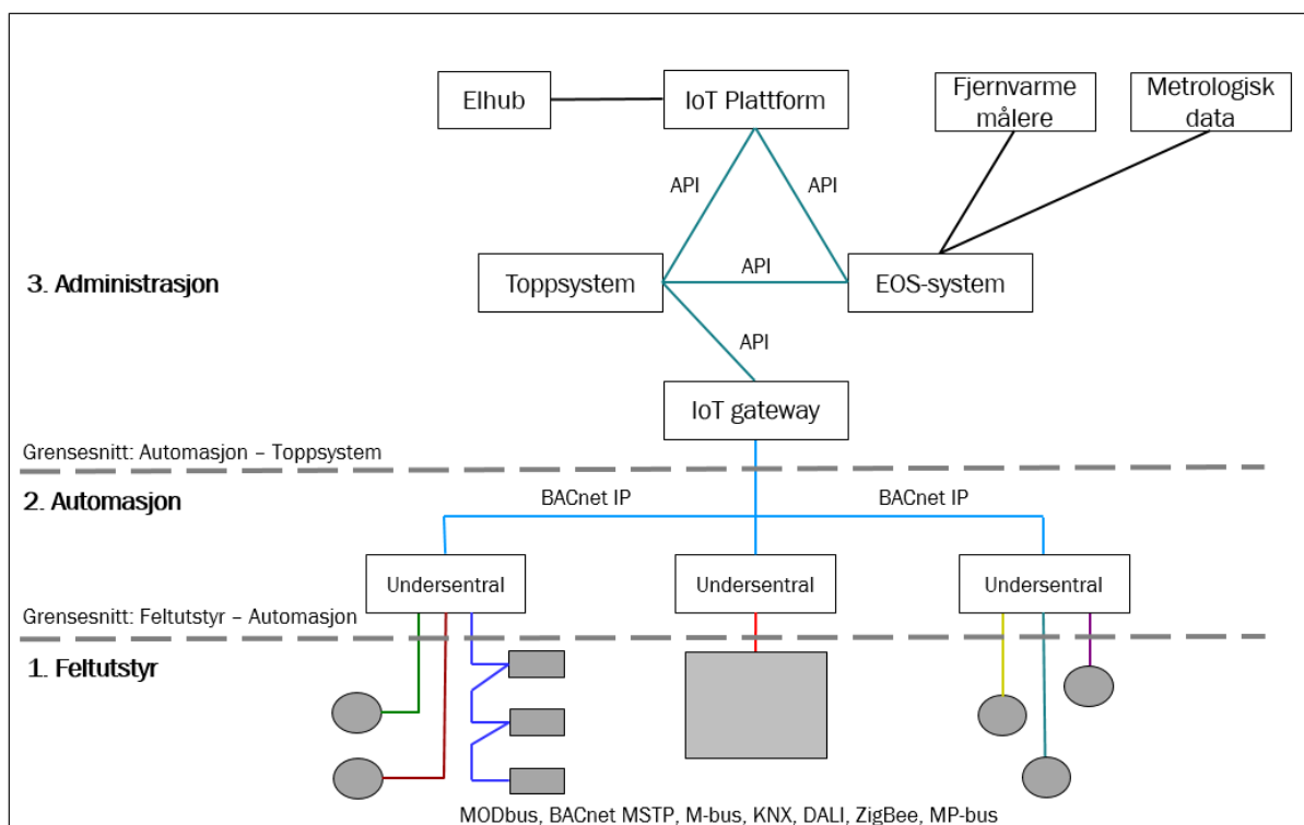
Figur 1: Prinsippsskisse for BAS og EOS arkitektur.
