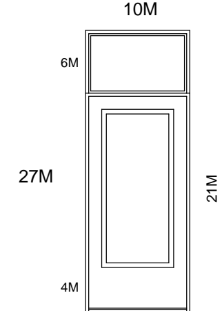
YD6 - 1 stk. H Inngangsdør med gl. felt, isolert tettfelt, sparkeplate begge sider, Klargjort kortleser
