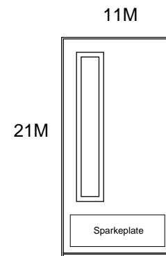
YD4 - 1 stk. H Inngangsdør med gl. felt, isolert tettfelt, sparkeplate begge sider, Klargjort for kortleser. Aut. døråpner
