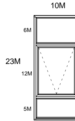
V5 - 3 stk. Tre - rams, fast karm, toppsving, solreflekterende glass
