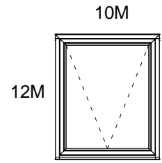
V2 - 3 stk. Ett rams, toppsving
