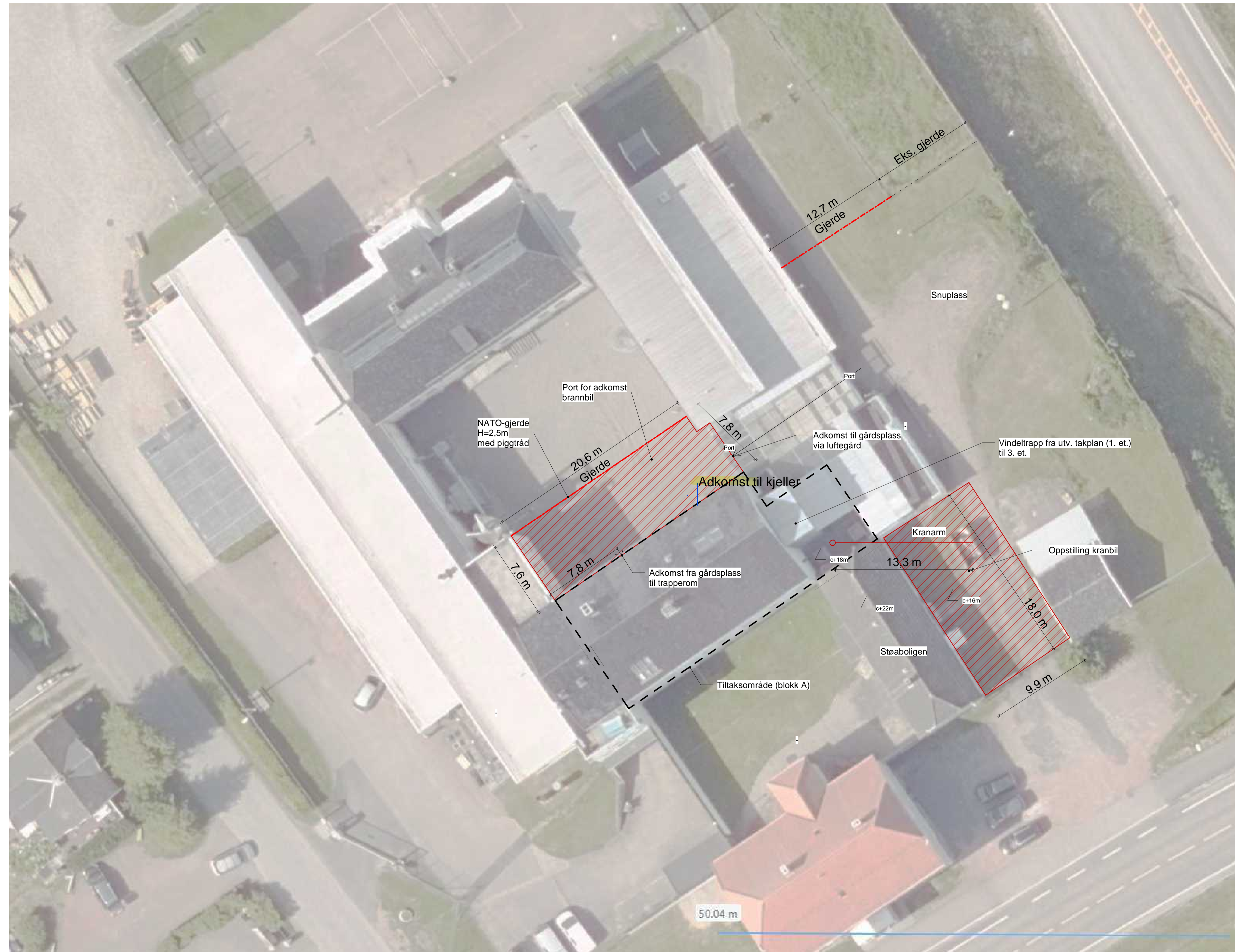
Riggplan 1 : 200
