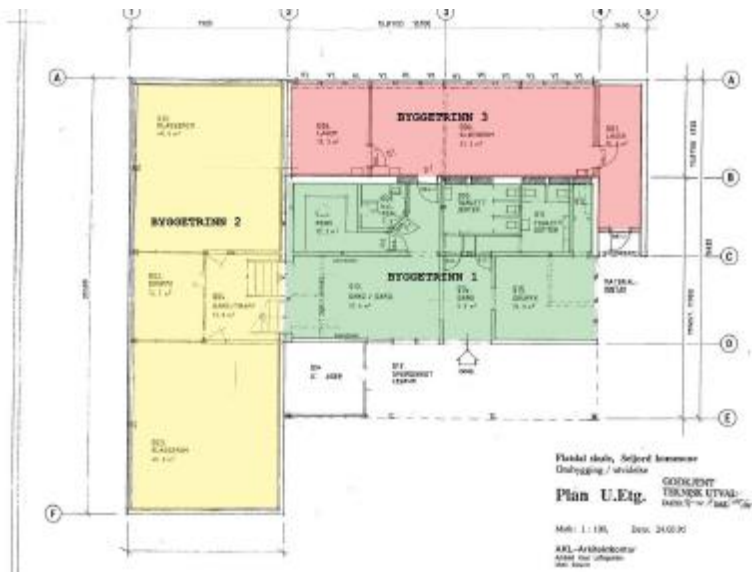
Figur 1 viser oversikt over dei ulike byggetrinna i plan U. Etg.
