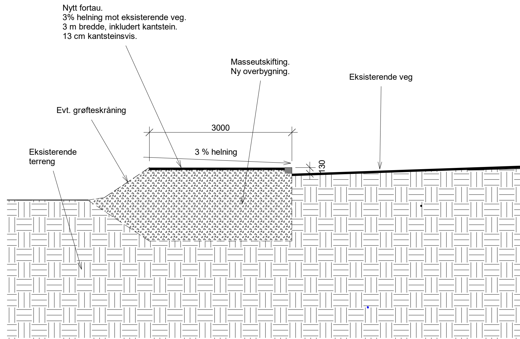
Prinsippsnitt 1 : 50
