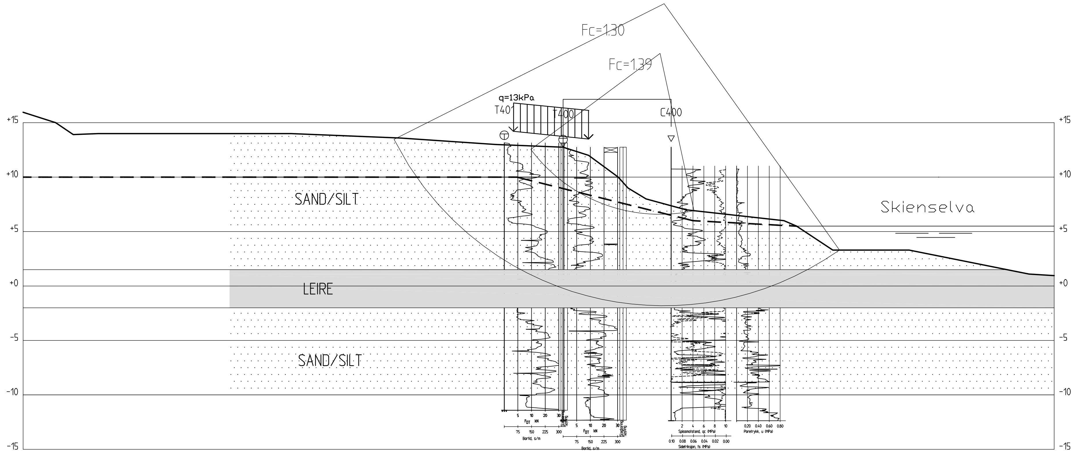
Profil A-A 1 : 200
