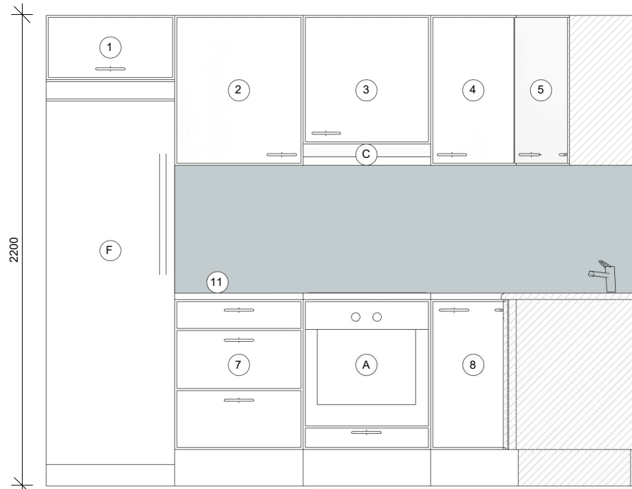
A 1 : 25
