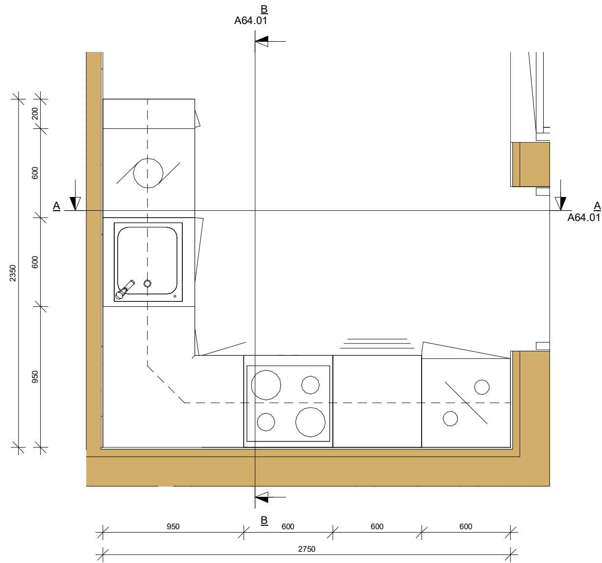
Kjøkken 1 : 25
