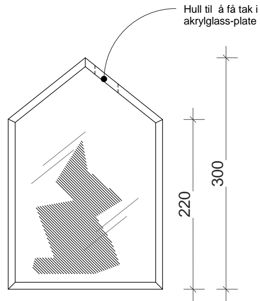
Oppriss
