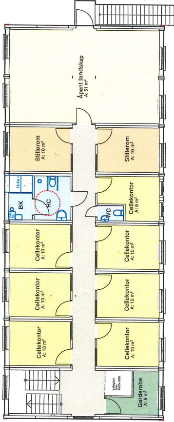
Andre etasje 1:150
