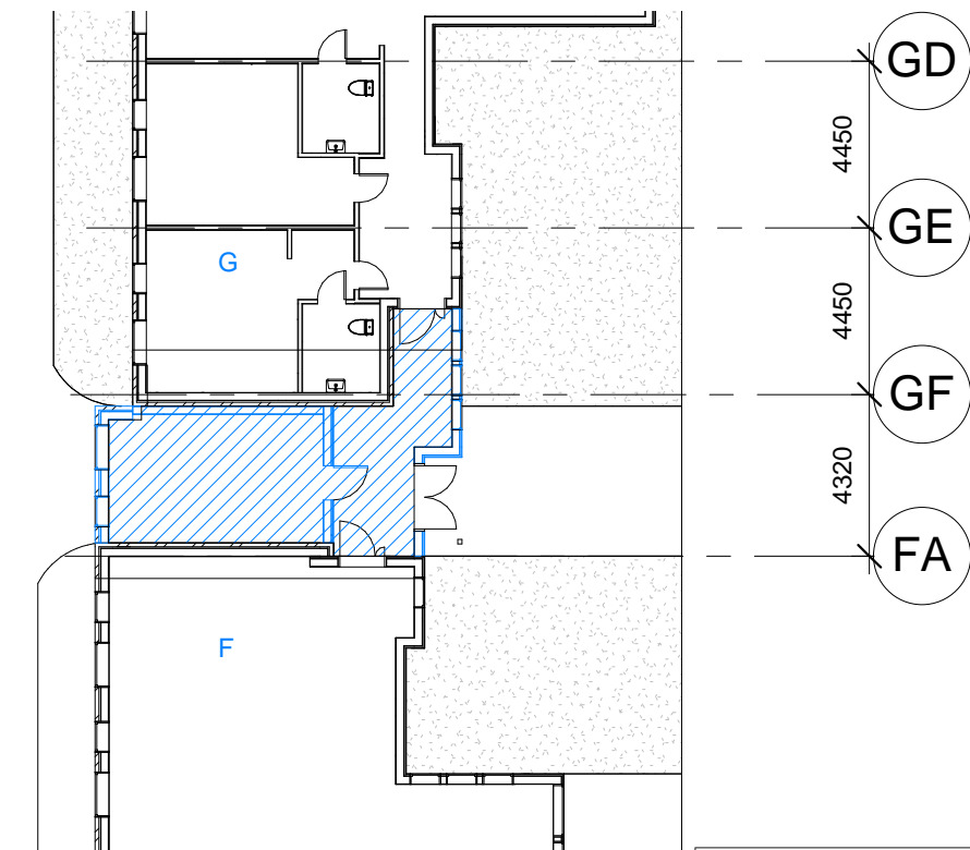
Utsnitt Bygg F og G 1:200
