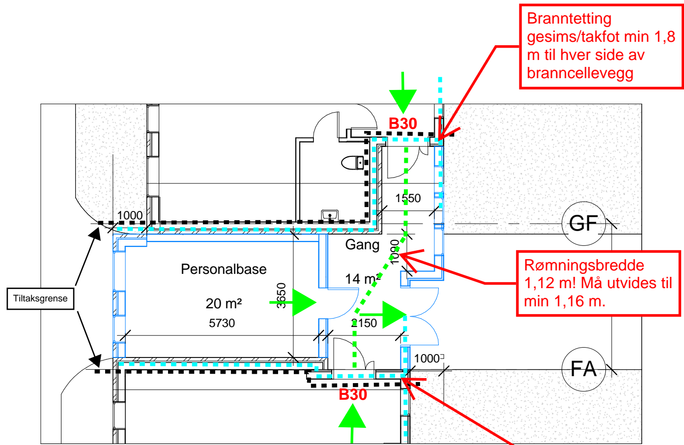
Planforslag tilbygg 1:100
