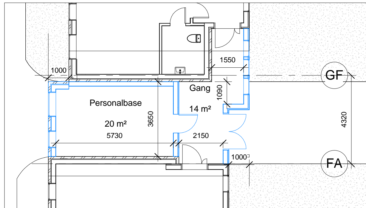
Planforslag tilbygg 1:100
