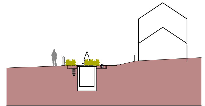
Snitt 1 : 200
