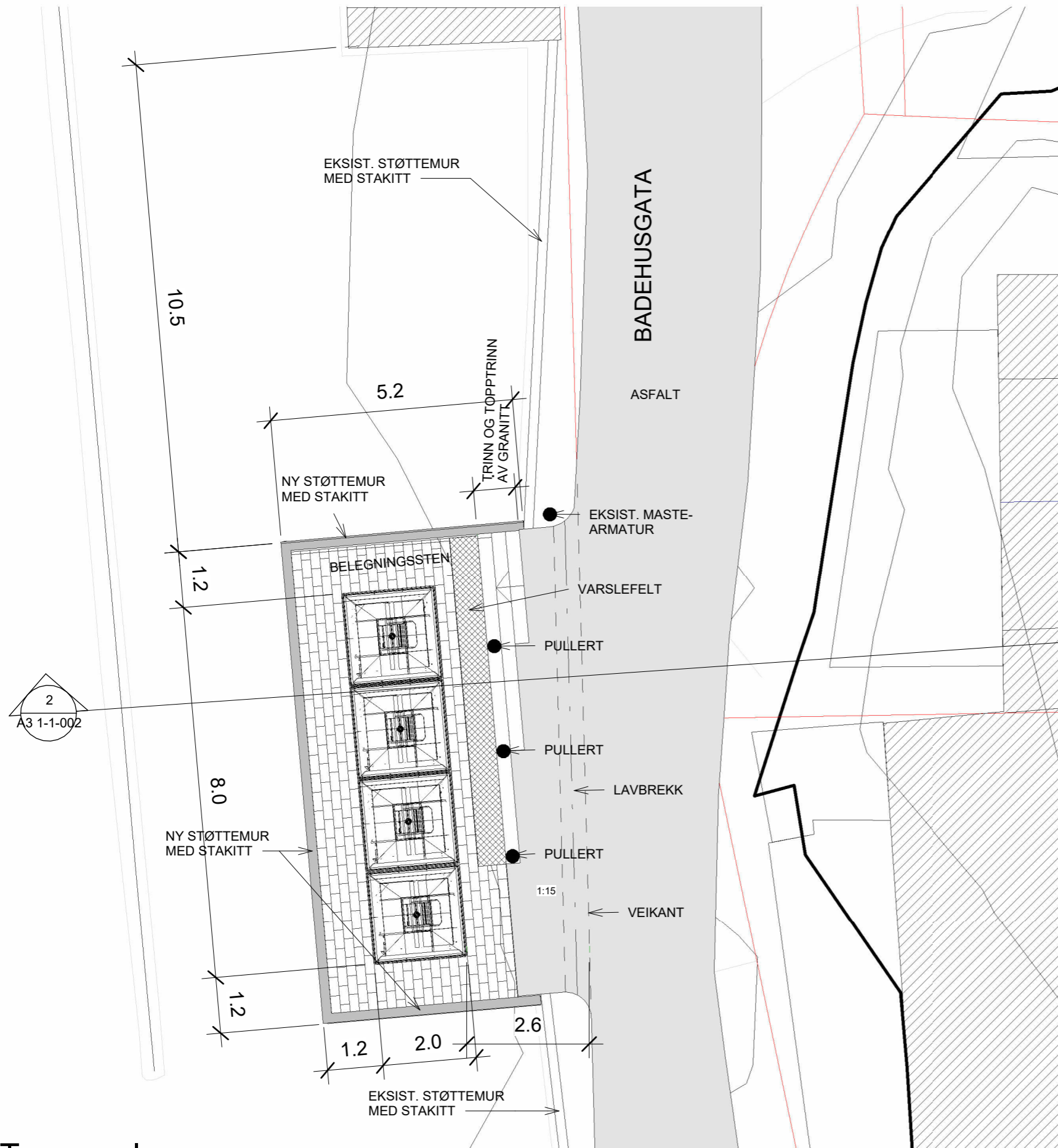
Terrengplan 1 : 100
