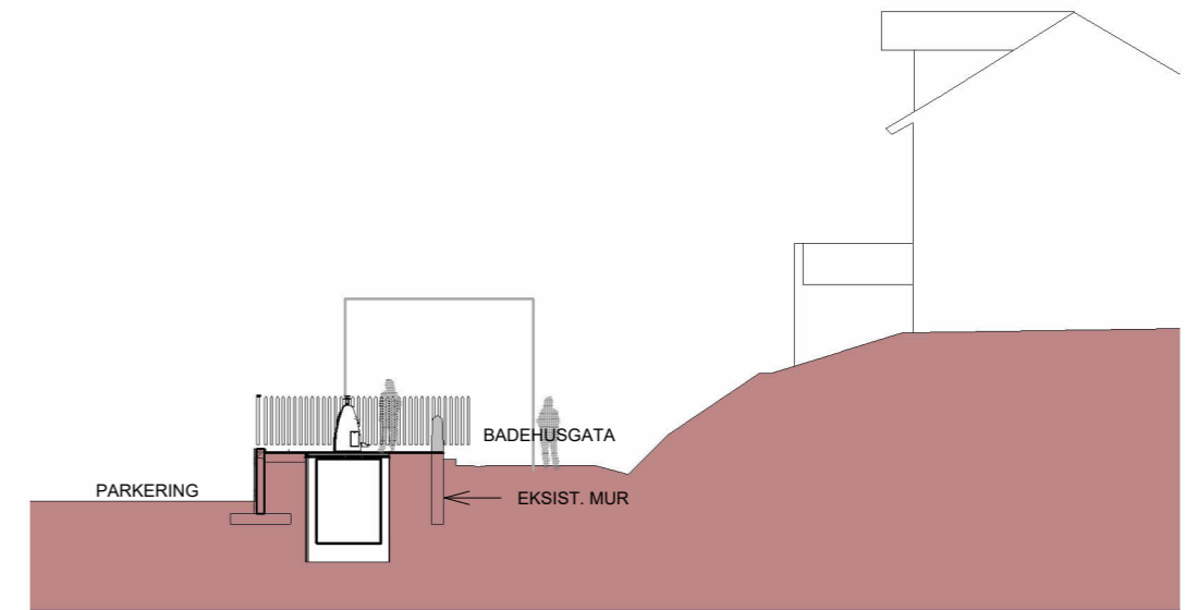
Snitt 1 : 200
