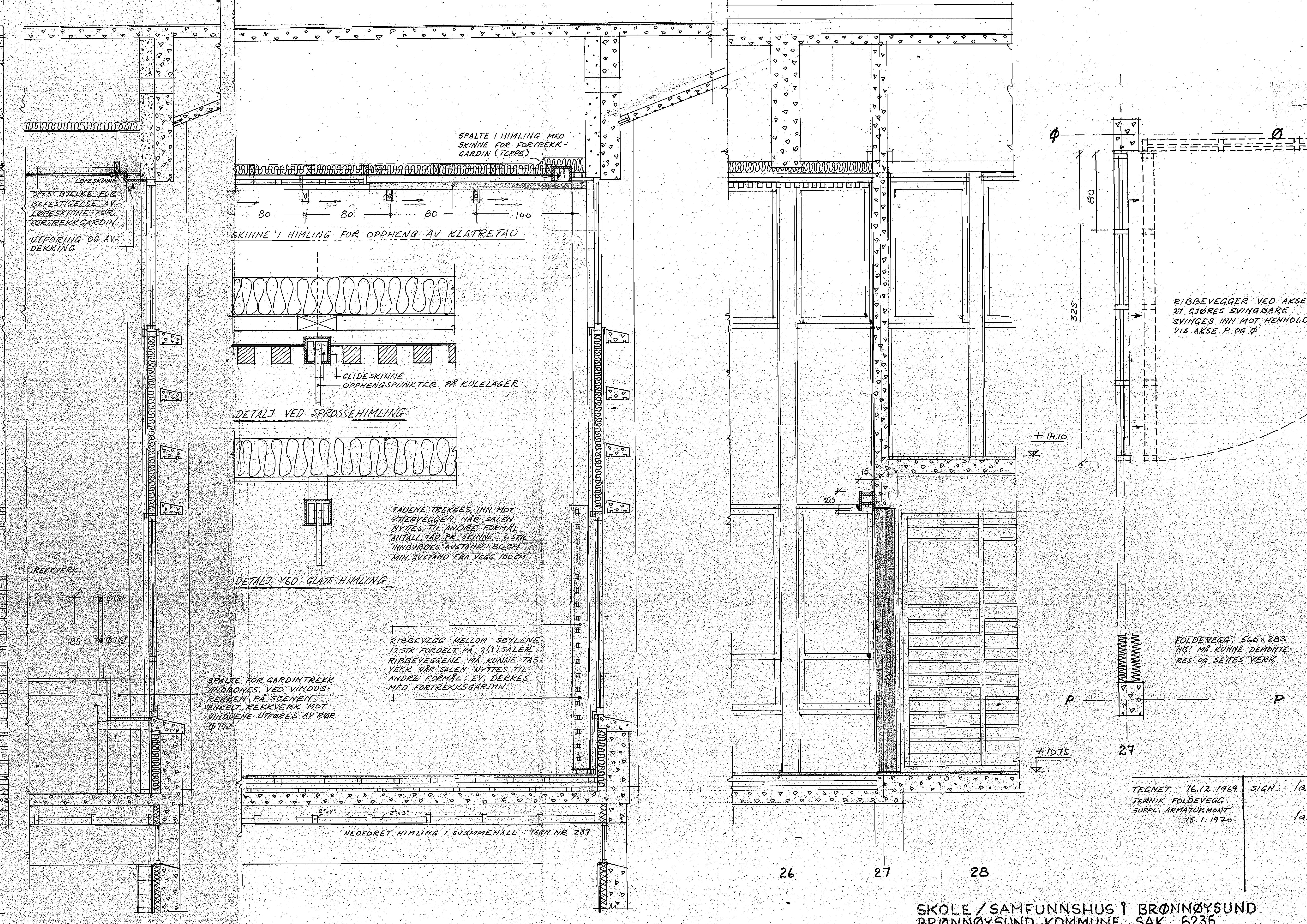
SNITT 3-3
