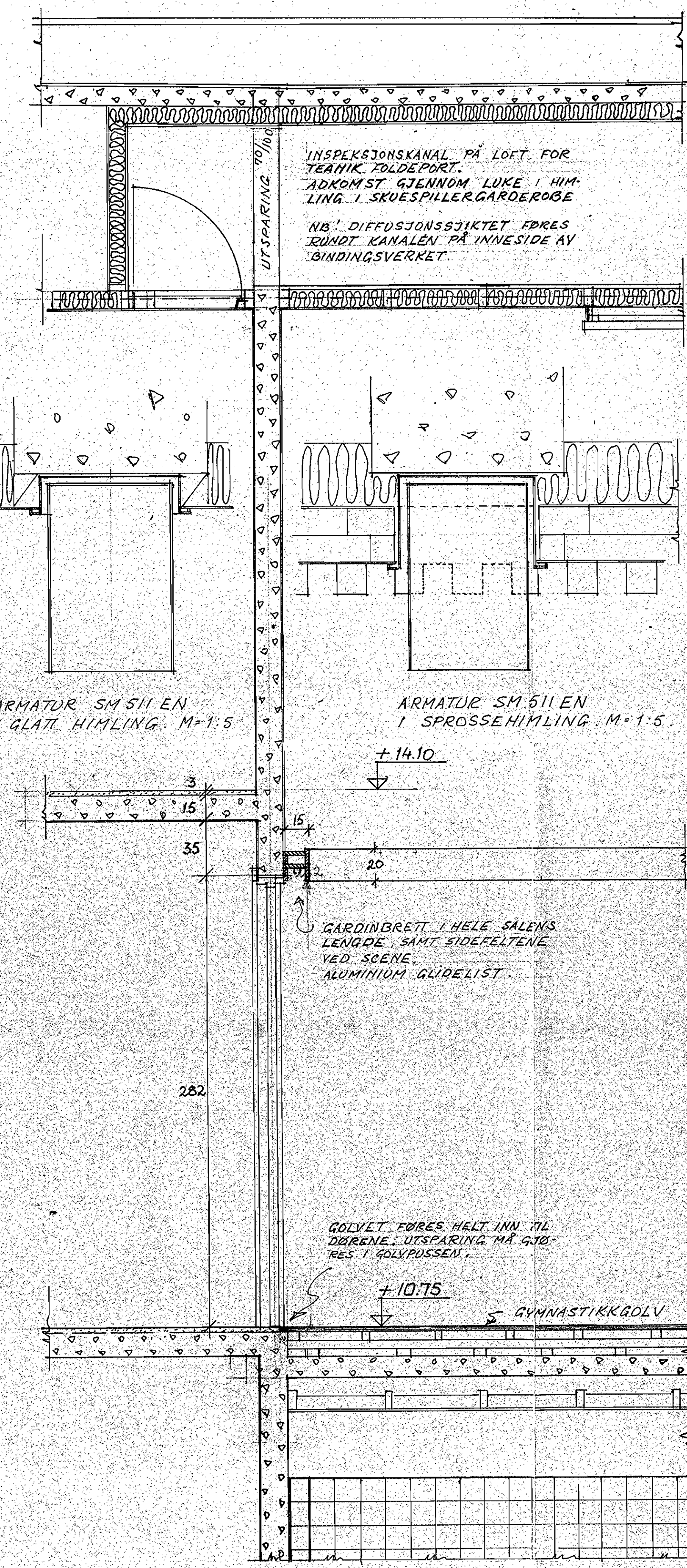
SNITT 16-16.
