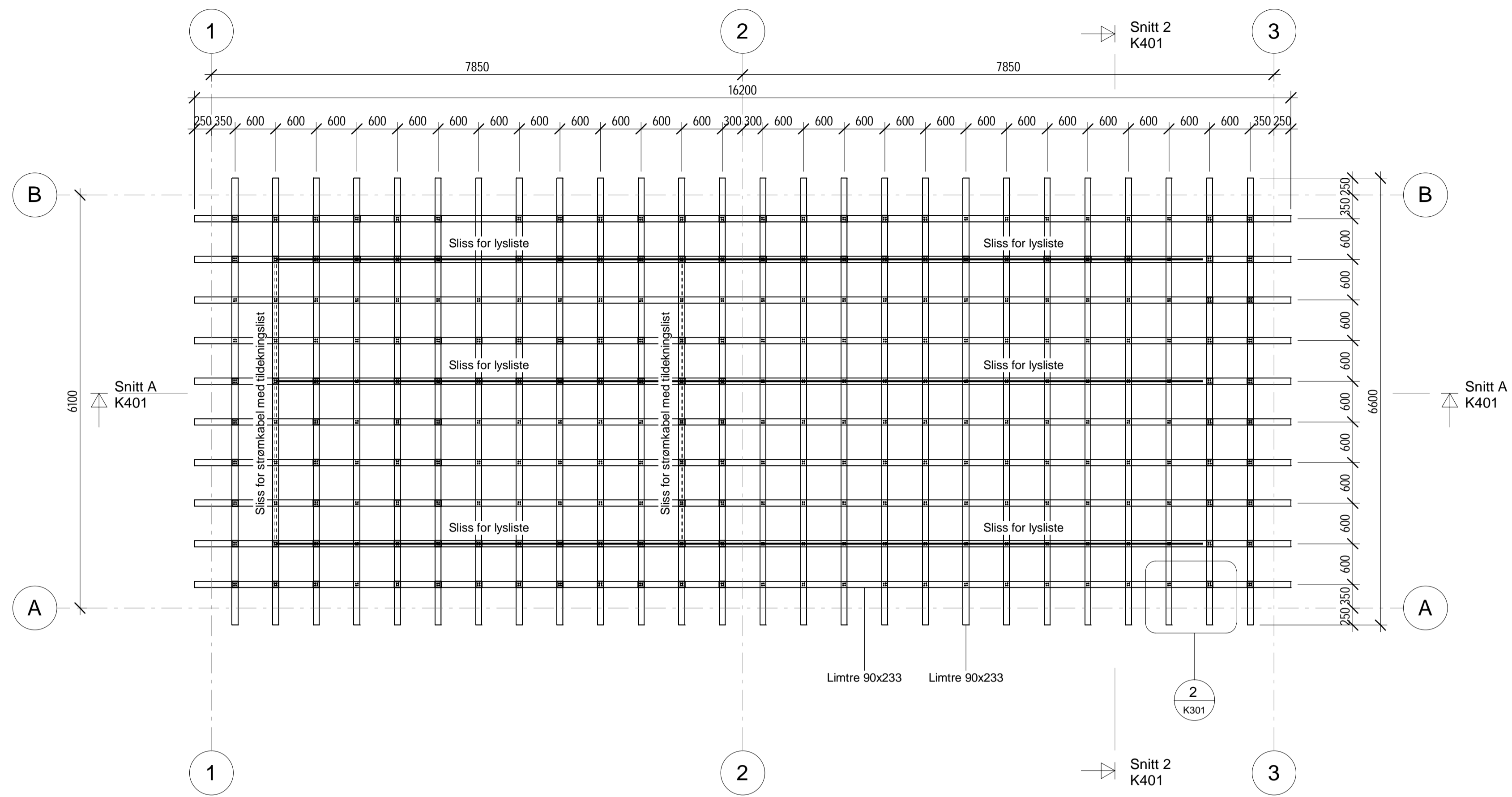
Bjelkeplan 1 : 50
