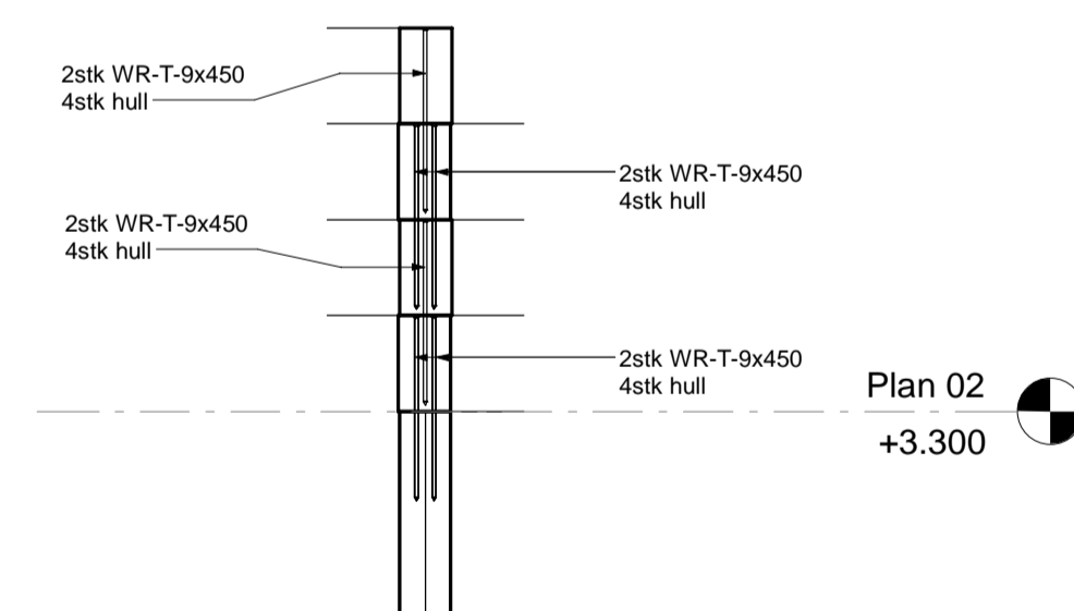
Skruer i bjelke-søylekryss 1 : 20
