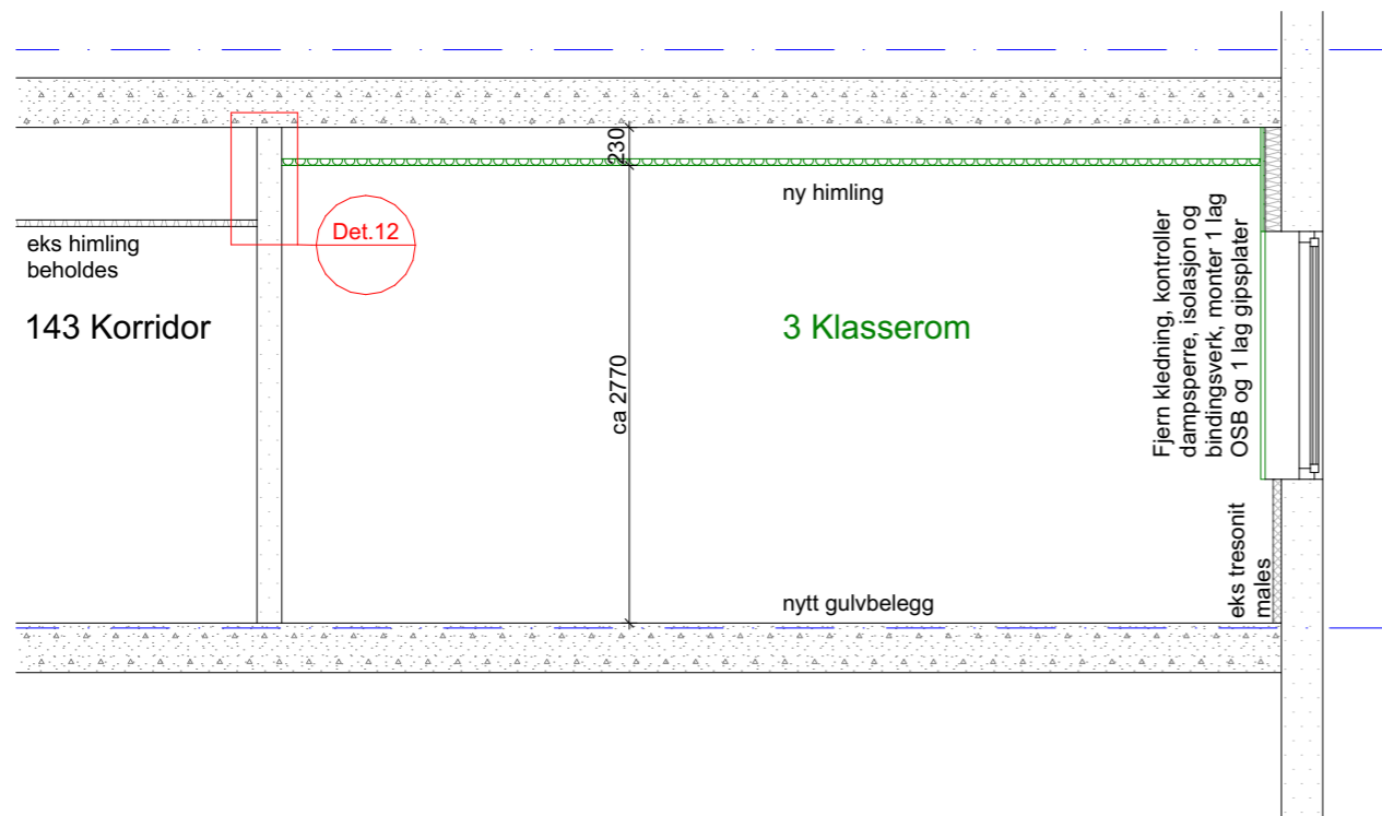
1:50 Snitt 3
