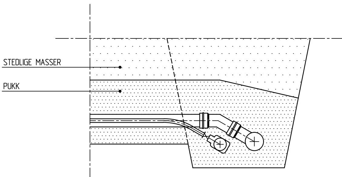
SNITT
