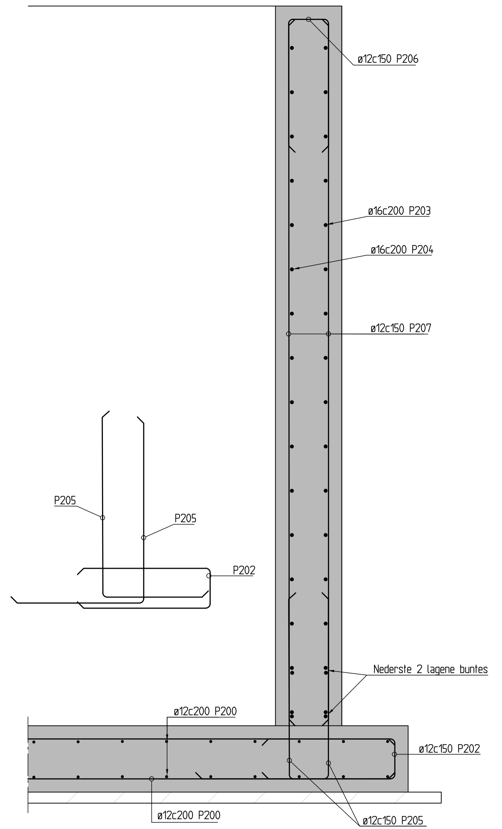
GENERELT SNITT 1:10
