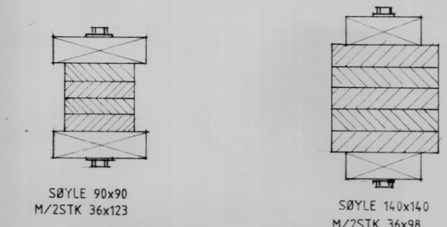
UTVENDIGE SØYLER 1:5
