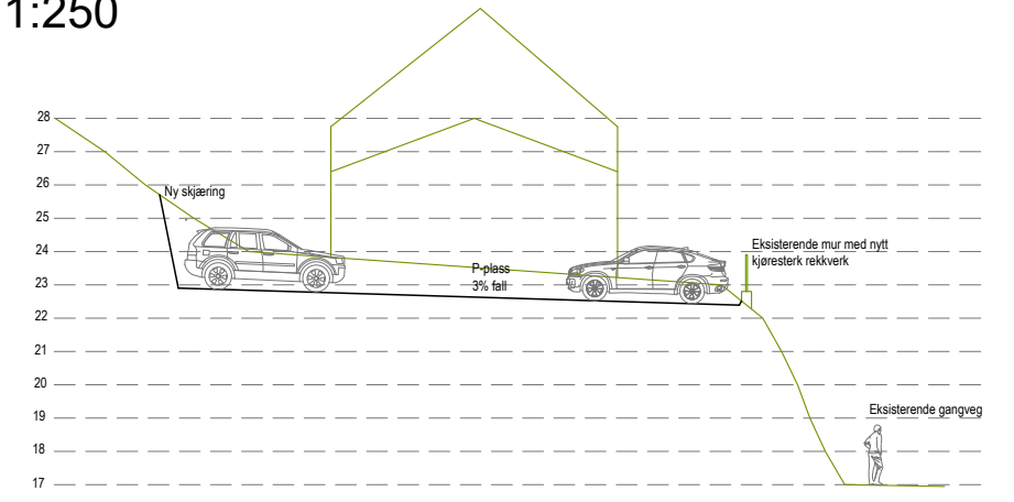
Snitt B 1:250
