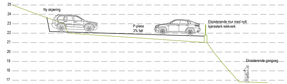
Snitt B 1:250
