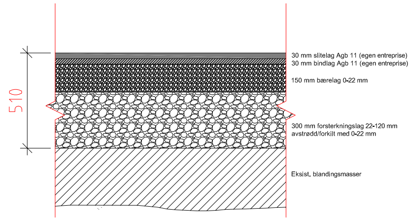
Overbygning asfaltert kjøreareal - område 2 og 4
