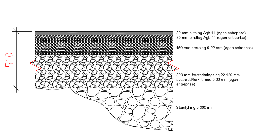
Overbygning asfaltert kjøreareal - område 1 og 3
