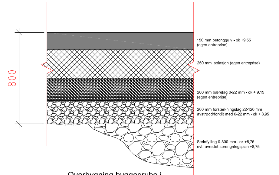
Overbygning byggegrube i område 1 og 3
