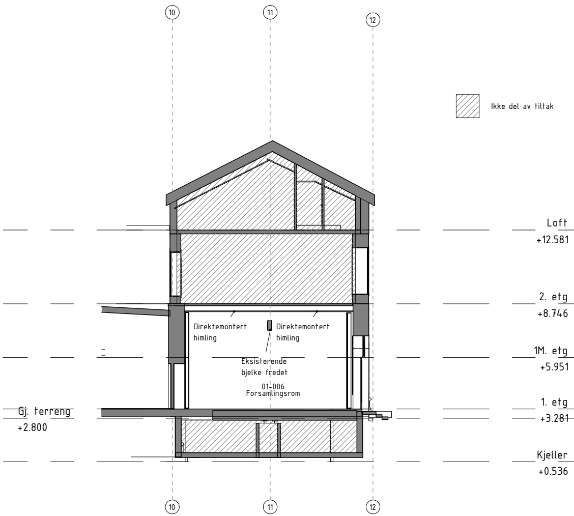
Snitt C-c, orienterende 1:200
