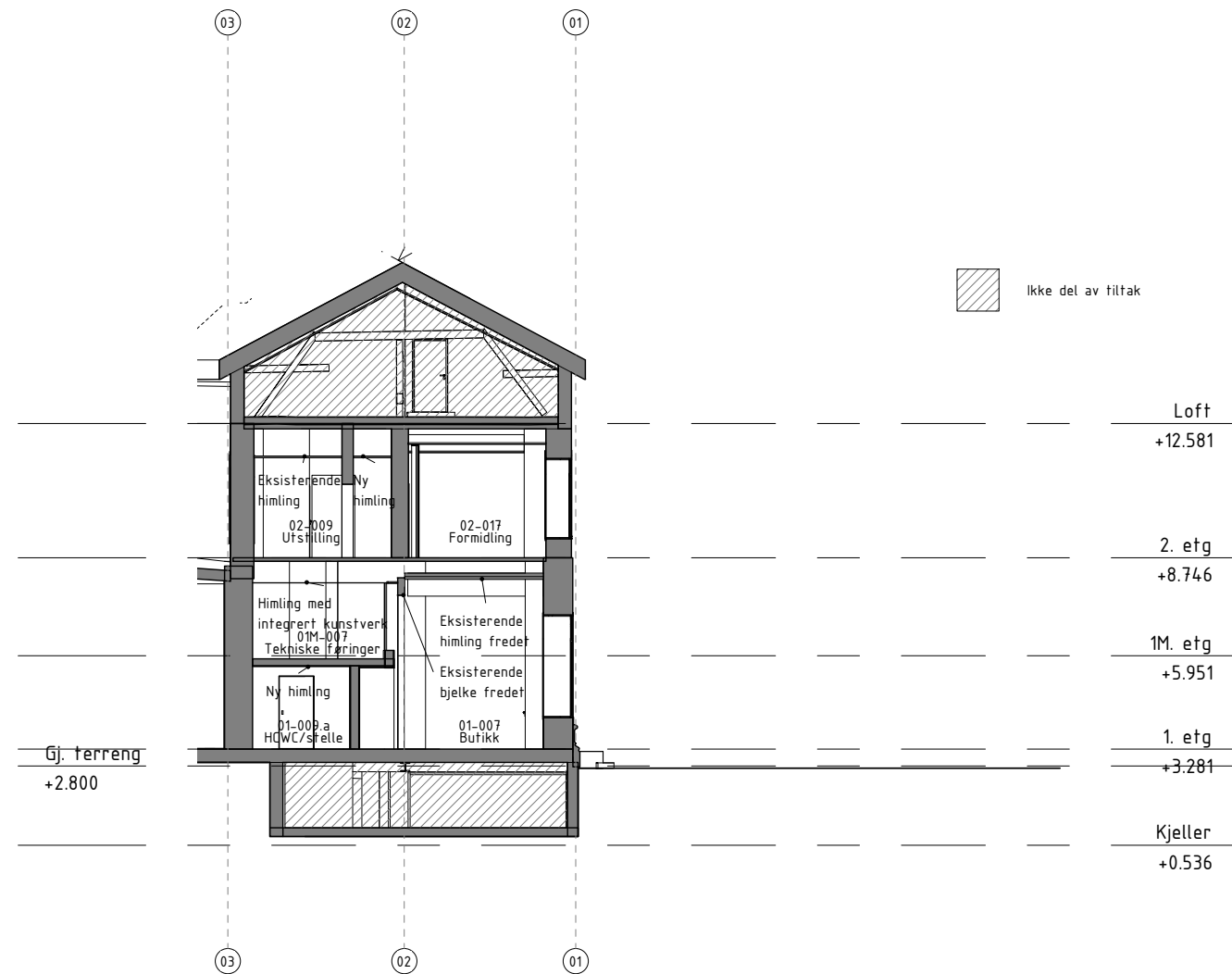
Snitt A-a, orienterende 1:200
