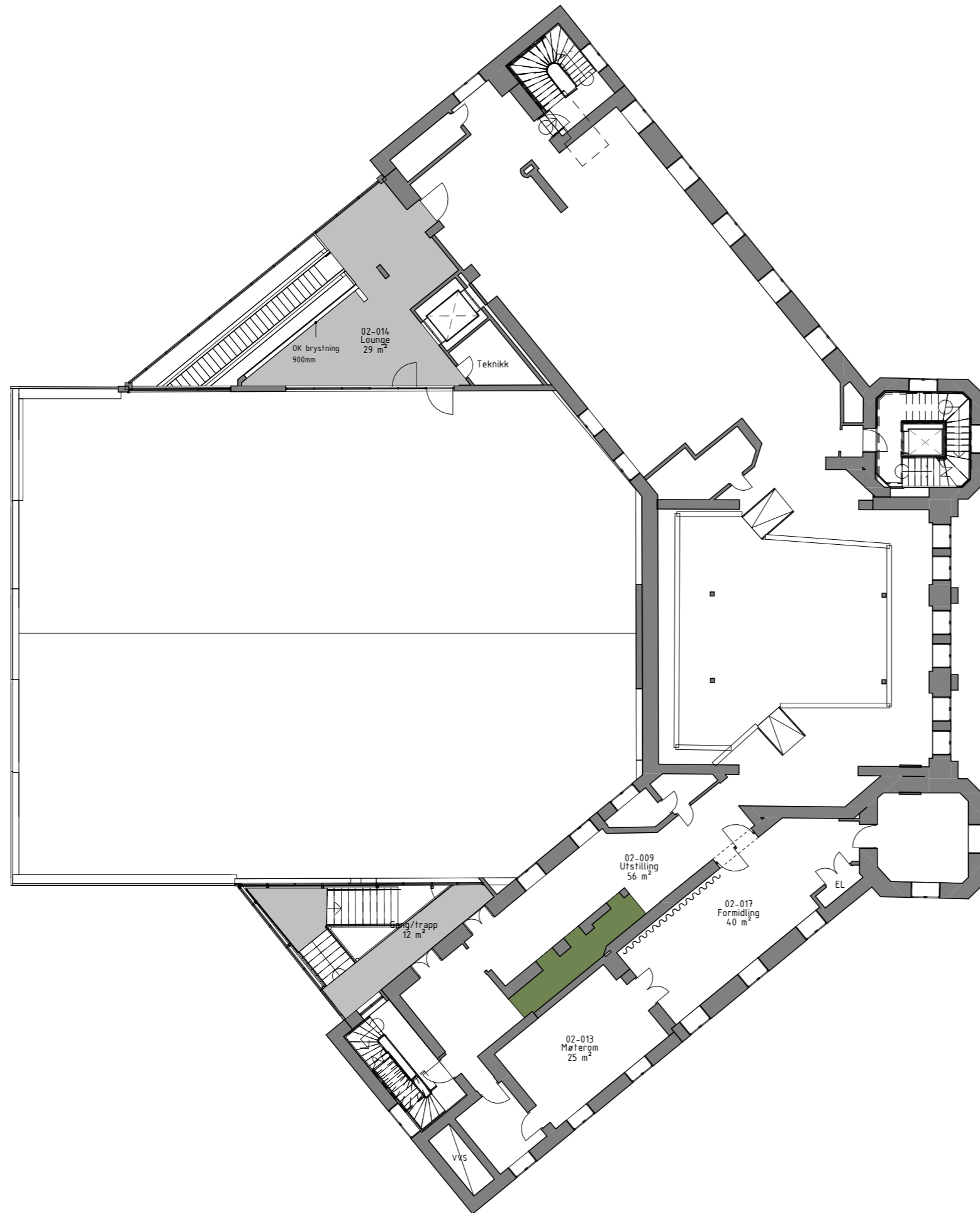
Gulvplan 2.etg 1 : 200
