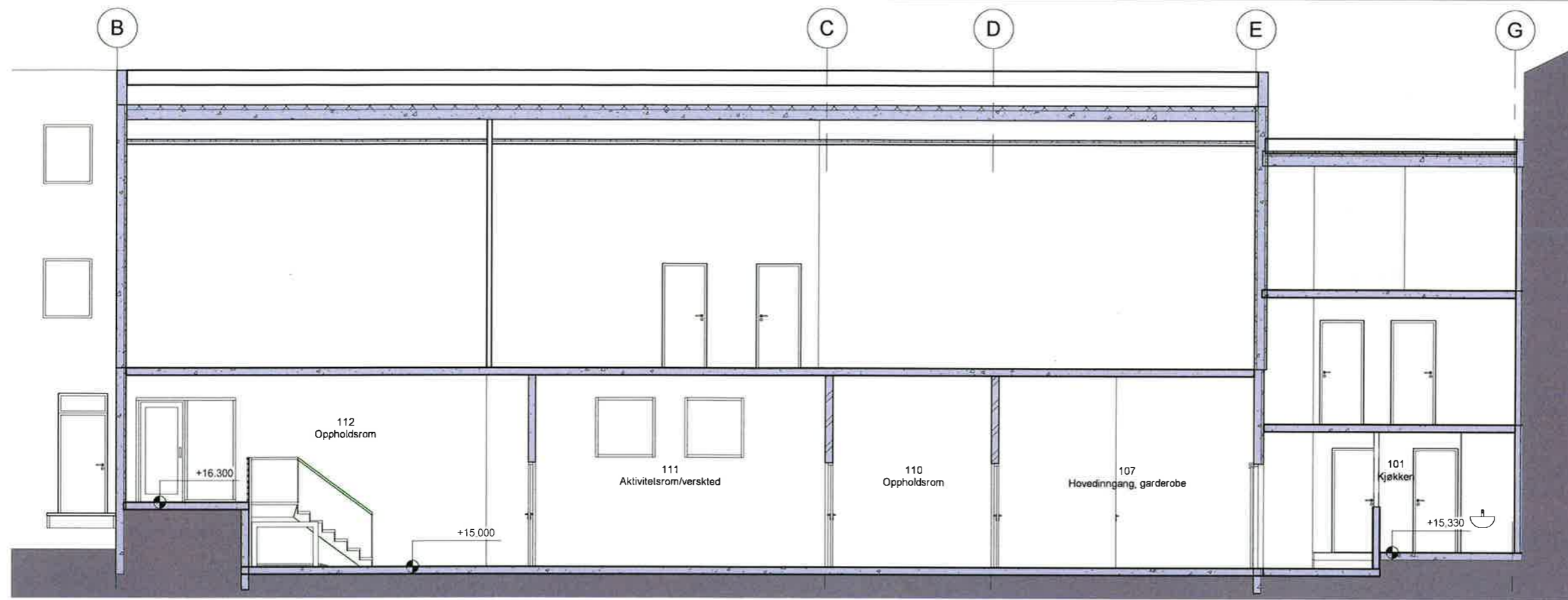
1 Langsnitt 1 : 100
