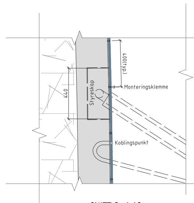
SNITT C - 1:10
