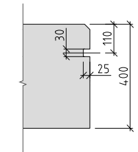
SNITT B - 1:10 IN052
