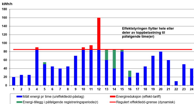
Figur 2. Eksempel på styring av 4 tilfeldige maksimalbelastninger ila. et døgn.
