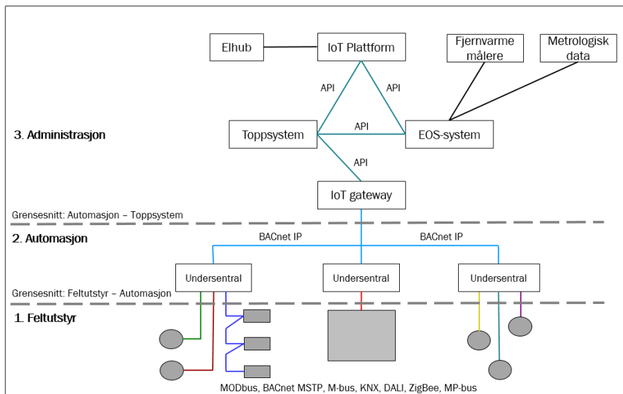
Figur 1: Prinsippskisse for BAS og EOS arkitektur.
