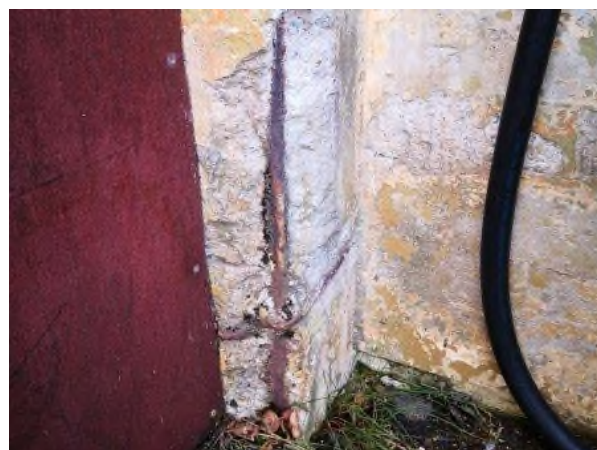
Figur 8: Synlig armering grunnmur
