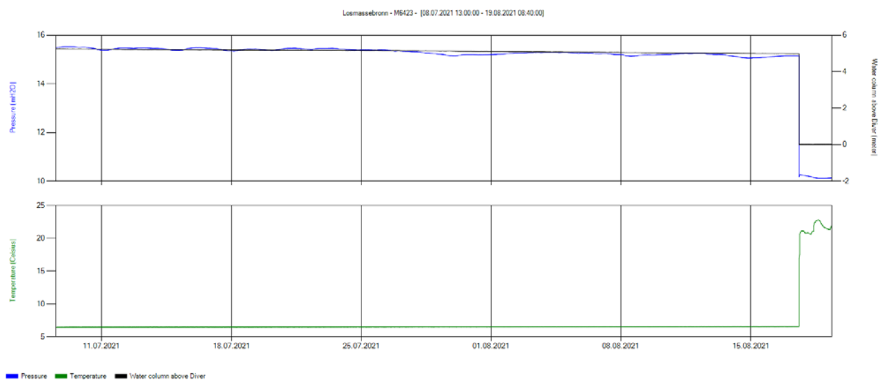
Figur 4-4 Målinger av grunnvannsnivå og temperatur i løsmassebrønnen, P31, sommer 2021.
