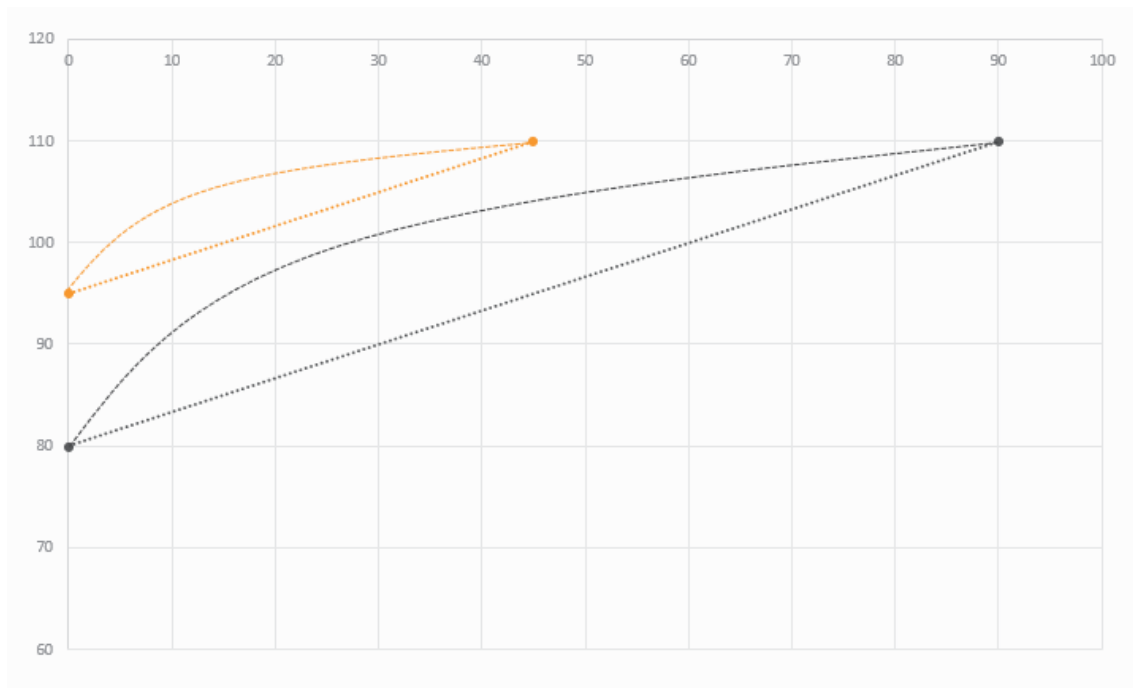
Figur 4-8: Graf viser en senkningskurve i distanse fra byggegrop (null), i lineær (overestimert) senkning og omtrentlig senkningskurve fra byggegrop basert på beregningene gjort på influensområde på bunnmorene. Stiplet oransje og stiplet sort linje viser senkningskurve med influensområde for henholdsvis 45 og 90 meter.
