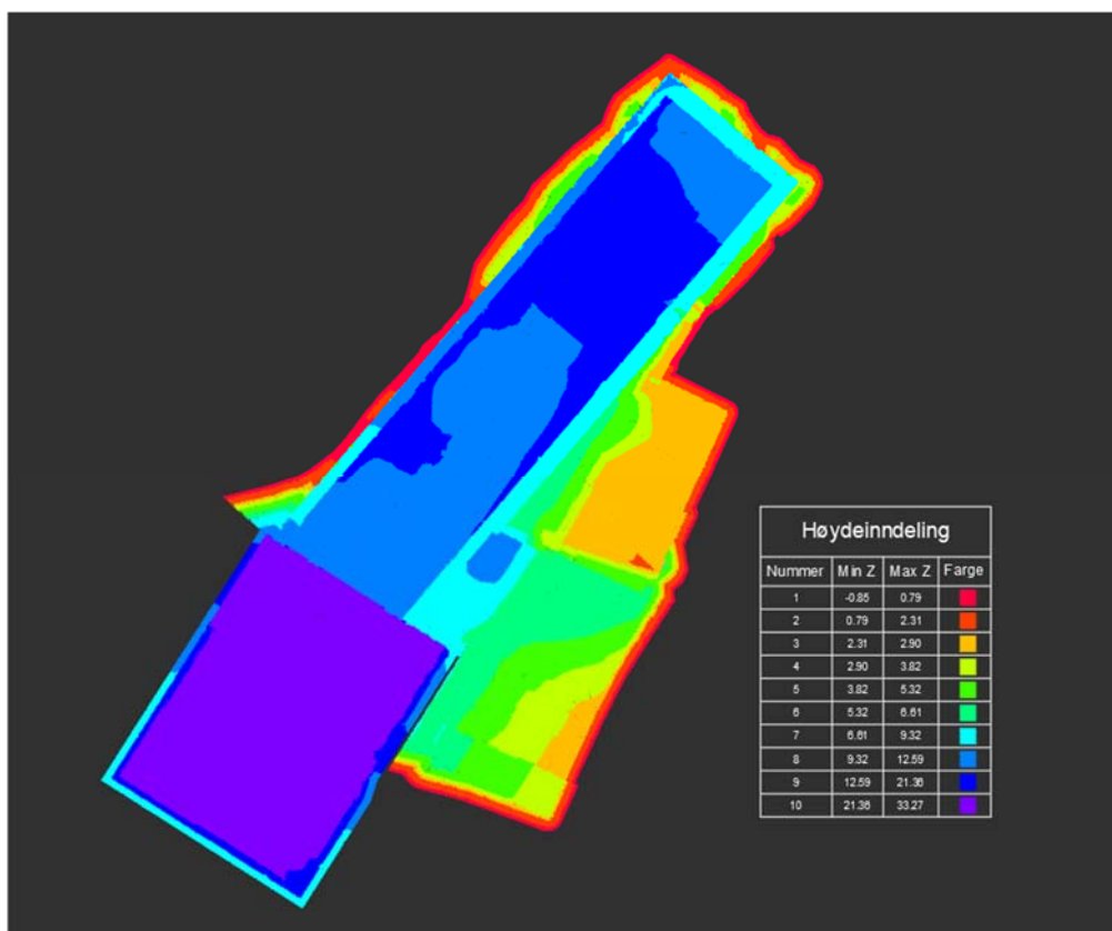
Figur 1-4: BIM-modell som viser byggegrop med prosjekterte dybder. Dybdene er fargekodet.
