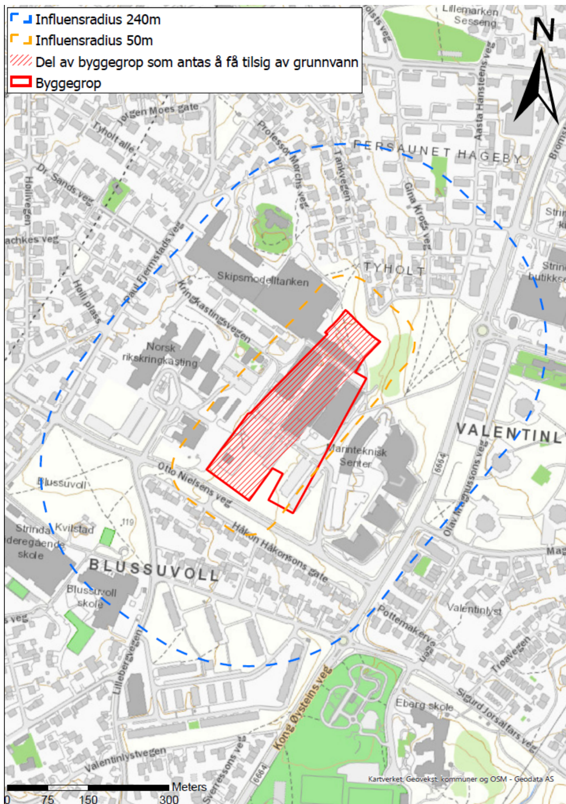
Figur 4-9: Delen av byggegropen hvor det skal graves til under grunnvannsstand og som antas kan ha påvirkning på hydrogeologien er skravert i rødt. Influensområder på 50 m (oransje) og 240 m (blått) er inkludert for å illustrere hvilke områder som beregningene indikerer at kan bli påvirket av prosjektgjennomføring.
