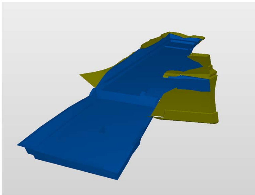
Figur 1-3: BIM-modell som viser prosjektert byggegrop, grønt viser til løsmasser og blått til berggrunn.
