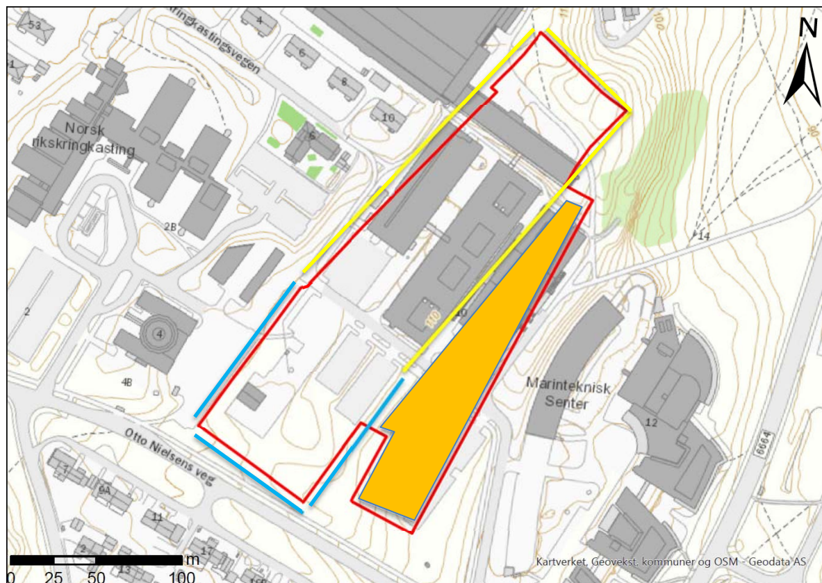
Figur 4-5: Utsnitt viser planlagt byggegrop markert med heltrukket rødt omriss. Sidene av byggegropen som er vurdert i forbindelse med innlekking er markert med blå og gul (hhv. 30 m og 15 m dyp byggegrop). Det oransje området markerer et område hvor det ikke er planlagt å grave mer enn 3 m under terreng. Det er ikke beregnet tilsig i dette området.
