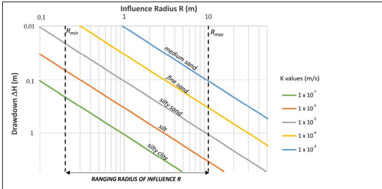
Figur 4-6: Sammenheng mellom senkning og influensområdet ved å benytte Sichardt's formel, gitt med ulike K-verdier (De Filippa et al., 2020), modifisert etter Fileccia, 2005.
