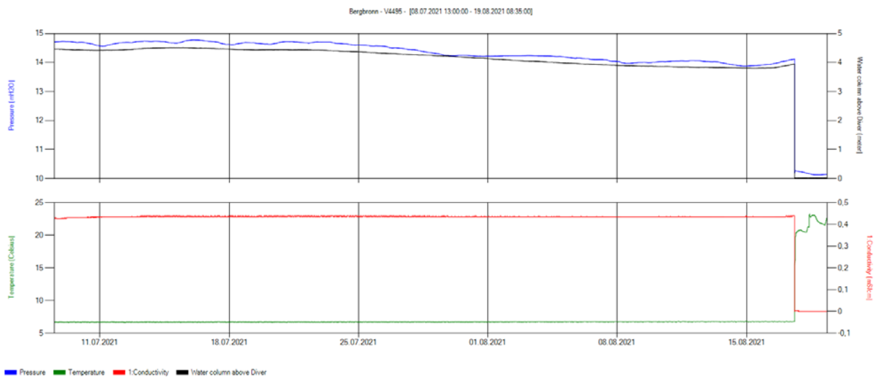
Figur 4-3 Målinger av grunnvannsnivå, temperatur og elektrisk konduktivitet i bergbrønnen, P1, sommer 2021.
