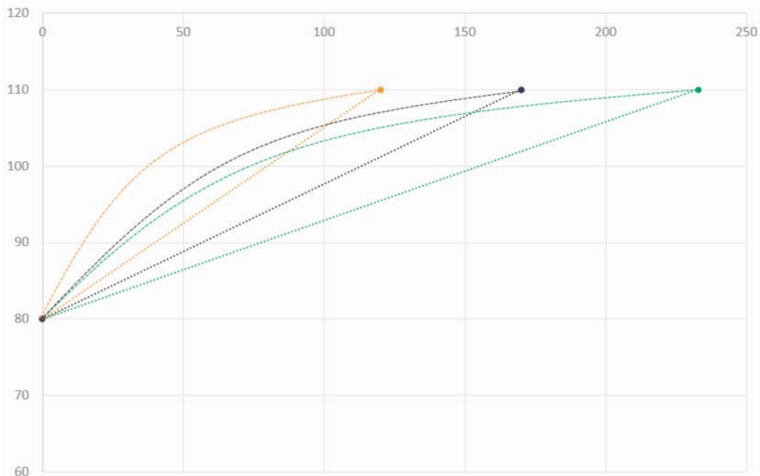
Figur 4-7: Graf viser en senkningskurve i distanse fra byggegrop (null på x-akse), i lineær (overestimert) senkning og skissert senkningskurve fra byggegrop basert på beregningene gjort på influensområde på berg. Stiplet oransje, stiplet sort og stiplet grønn linje viser senkningskurve med influensområde for henholdsvis 120, 170 og 233 meter.
