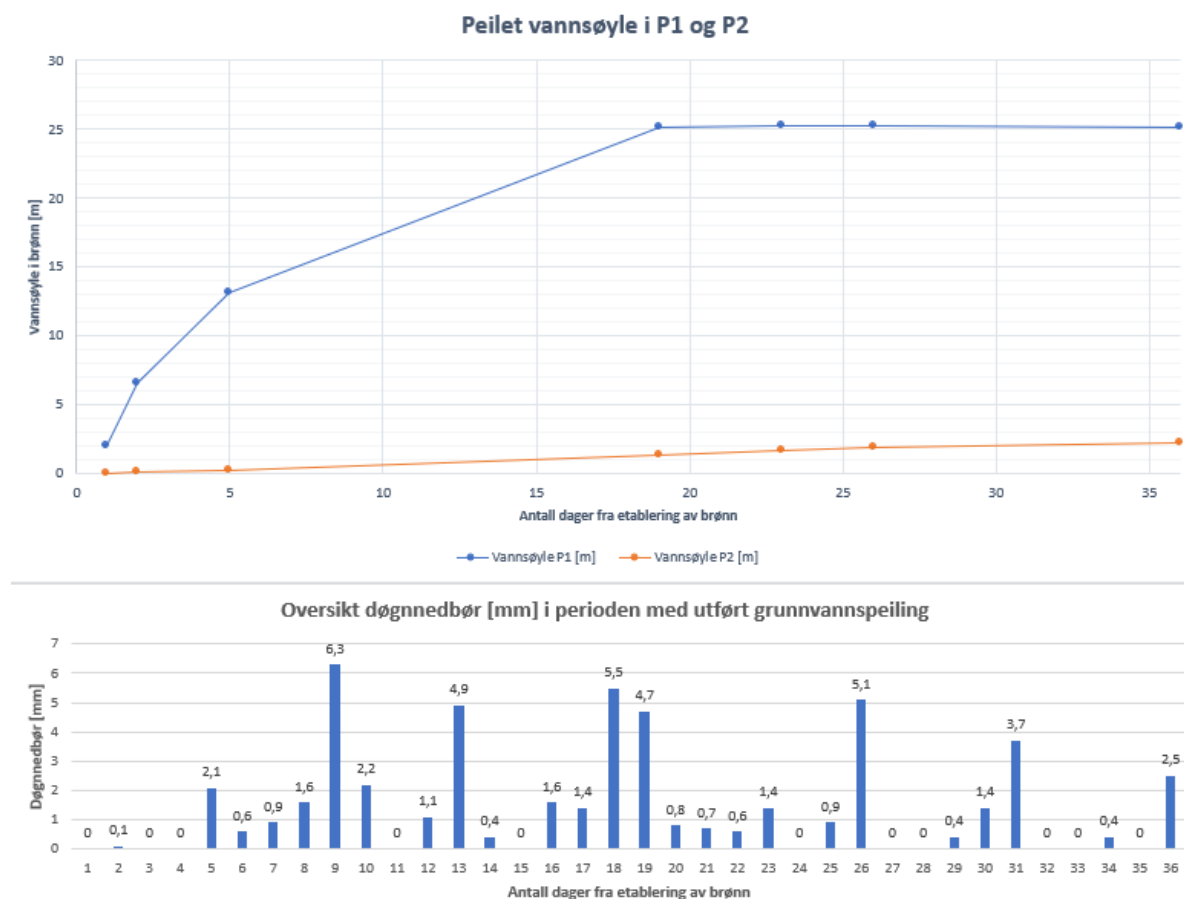
Figur 4-2 Presentasjon av hvordan vannshøyden i brønn P1 og P2 utvikler seg over tid basert på utført grunnvannspeiling
