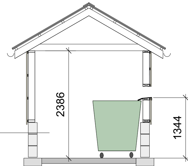
Snitt
