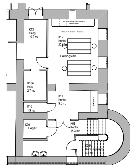
PLAN U 1:200 LÆRINGSLAB
