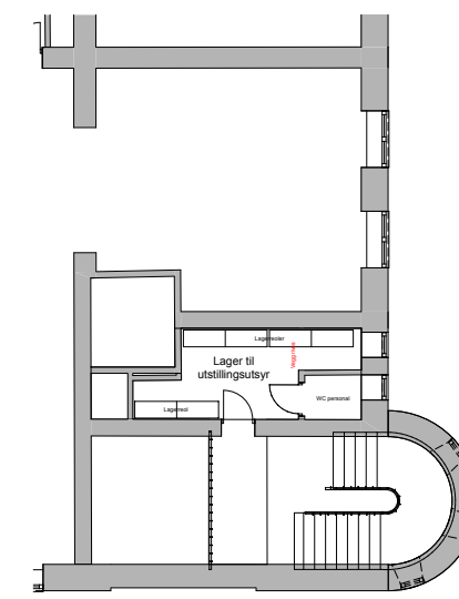
PLAN 1,5 1:200 LAGER
