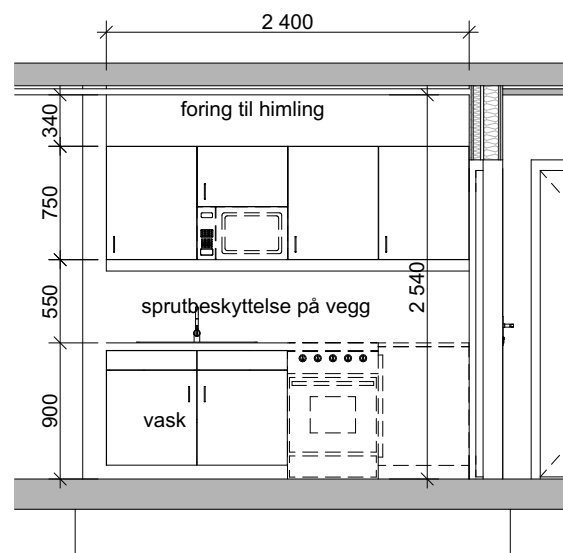
Leilighet 5: oppriss 1.50
