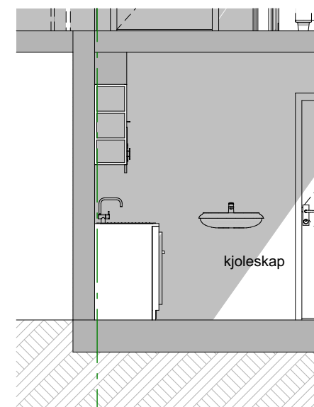
Allrom - kjøkken: oppriss 1.50
