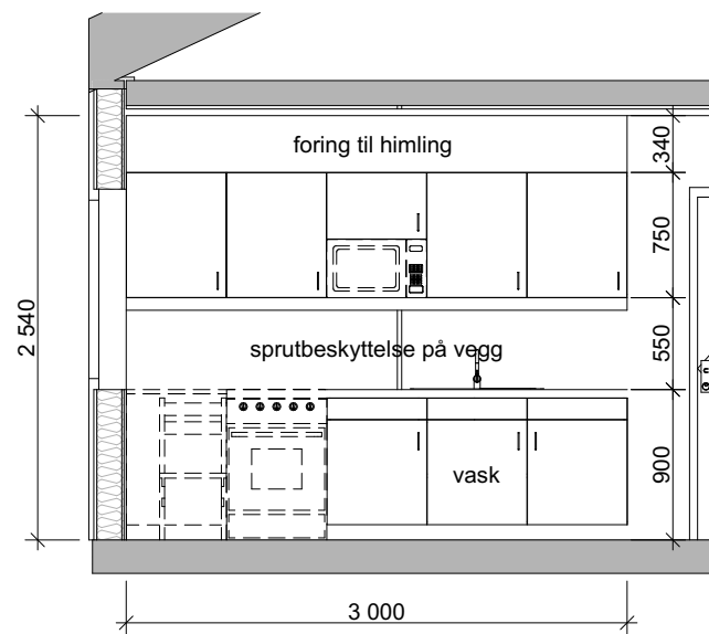
Leilighet 2: oppriss 1.50
