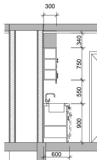
Leilighet 5: snitt 1.50
