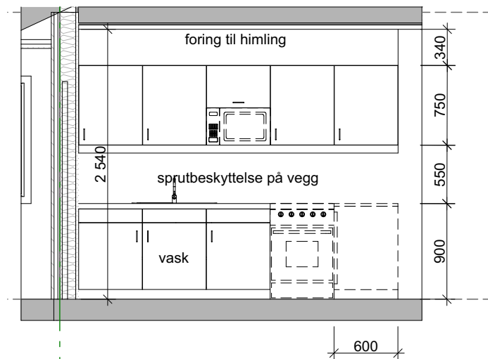
Leilighet 1: oppriss 1.50
