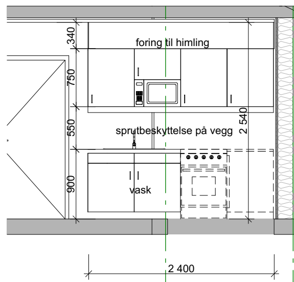
Leilighet 4: oppriss 1.50
