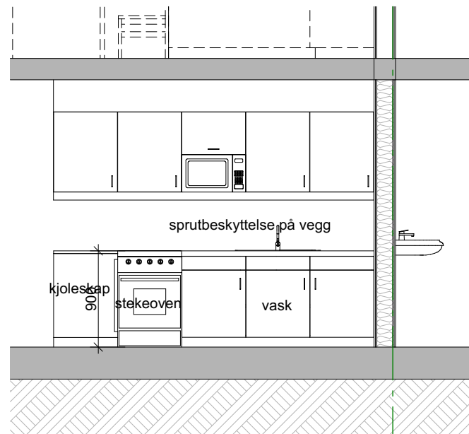
Allrom - kjøkken: oppriss 1.50
