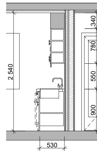
Leilighet 2: snitt 1.50
