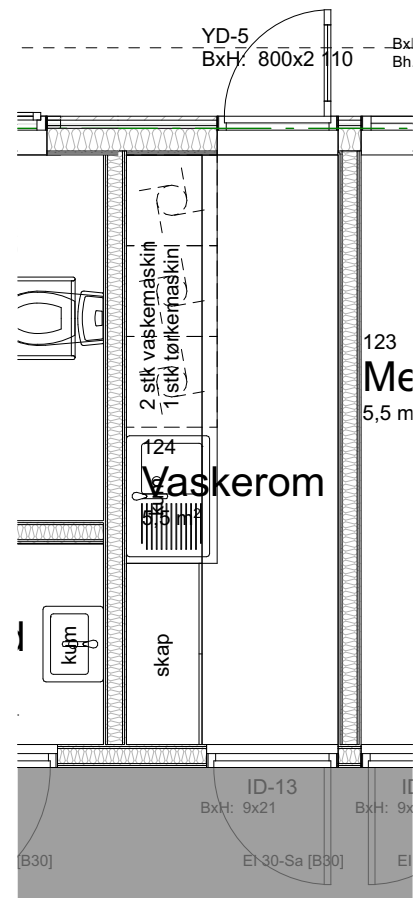
Vaskerom - Plan
