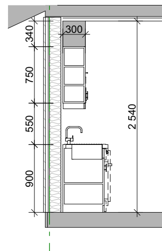
Leilighet 1: snitt 1.50
