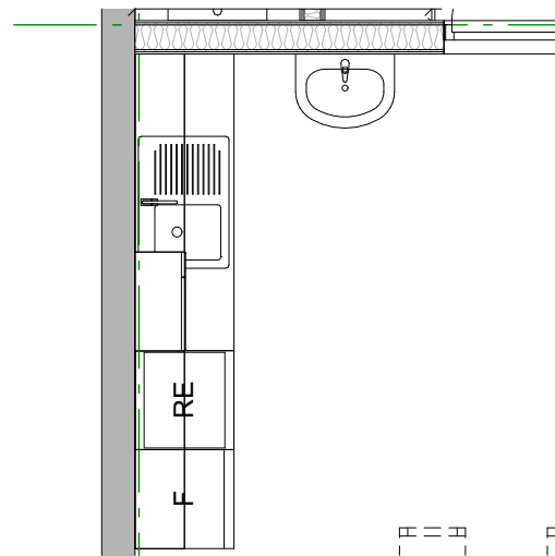
Allrom - kjøkken: plan 1.50
