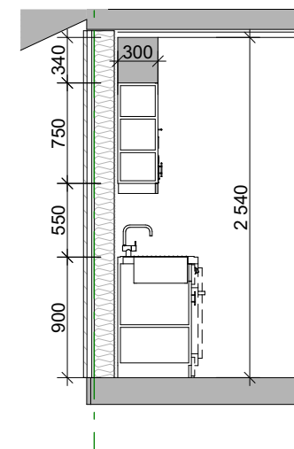
Leilighet 3: snitt 1.50
