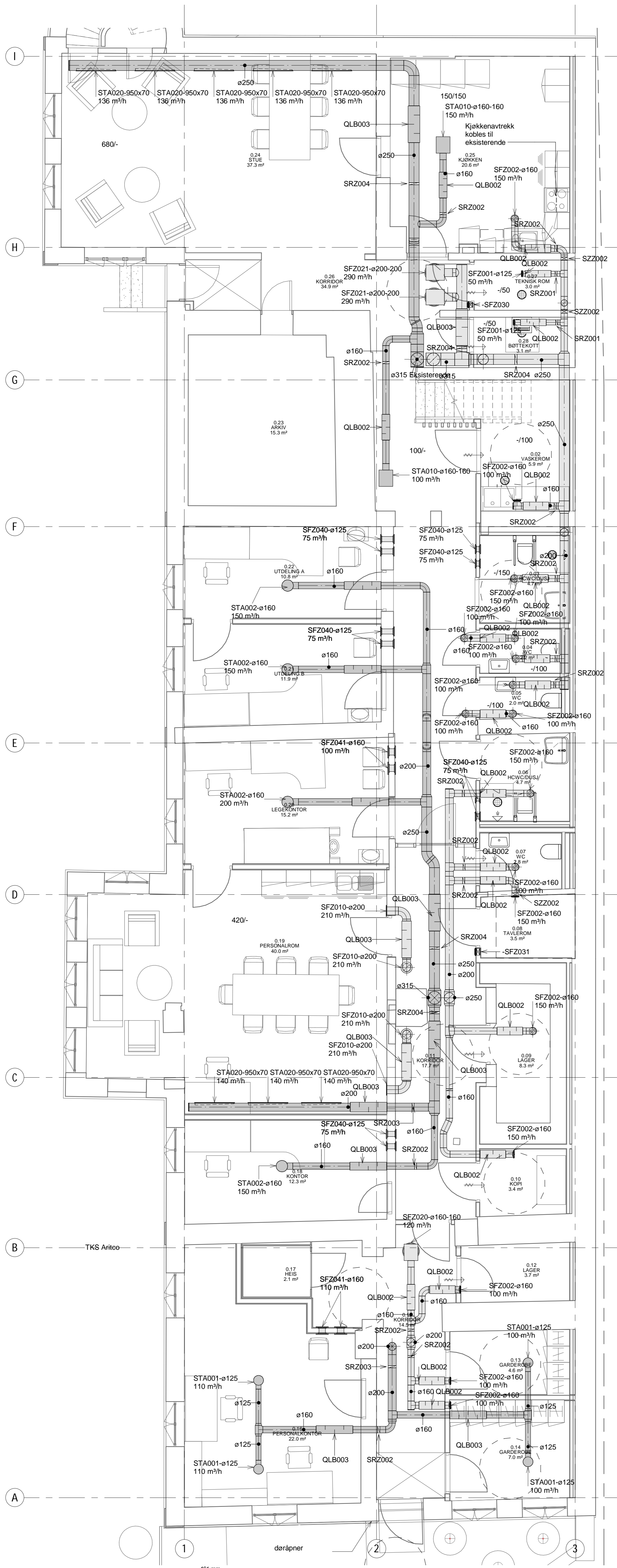
36 Venter/Rister Ventilasjonsanlegg U01
